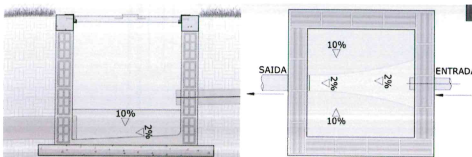
Modelo caixa de inspeção
