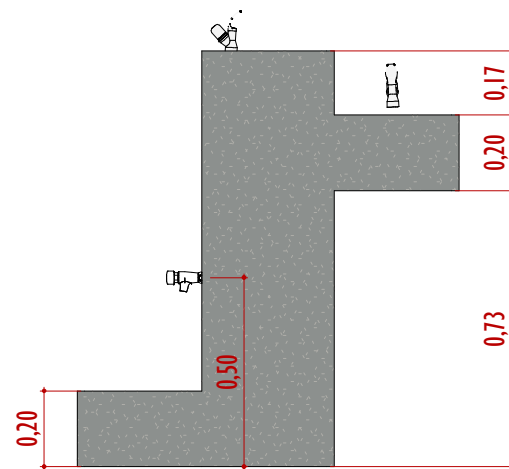
4 BEBEDOURO - ELEVÇÃO FRONTAL 1 : 20
