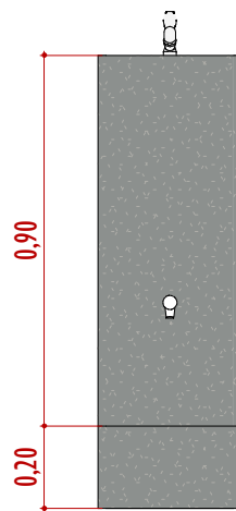
5 BEBEDOURO - ELEVÇÃO ESQUERDA 1 : 20
