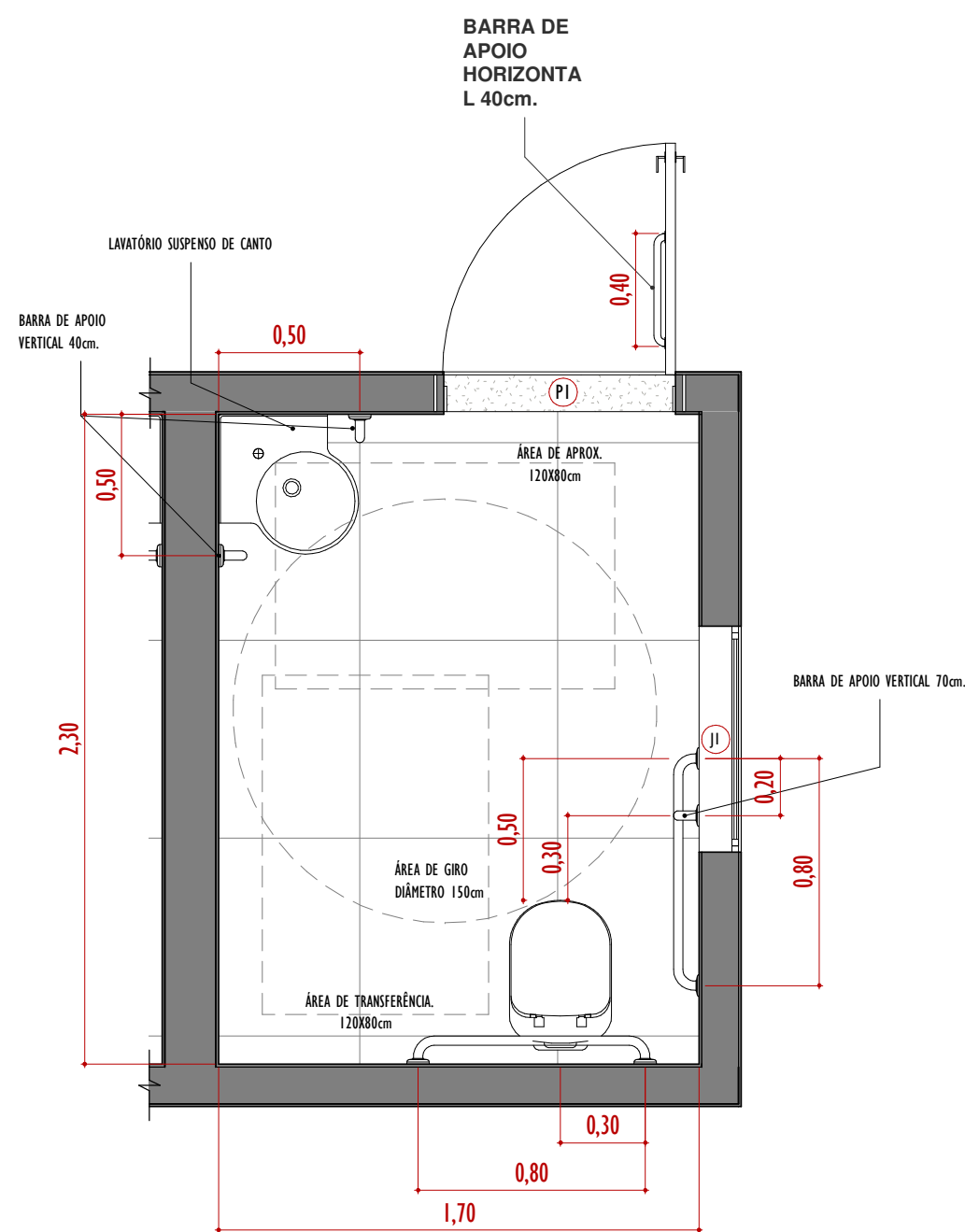
1 DET. ÁREA MOLHADA - WC PcD MASC. 1 : 25
