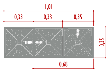
3 BEBEDOURO - VISTA SUPERIOR
