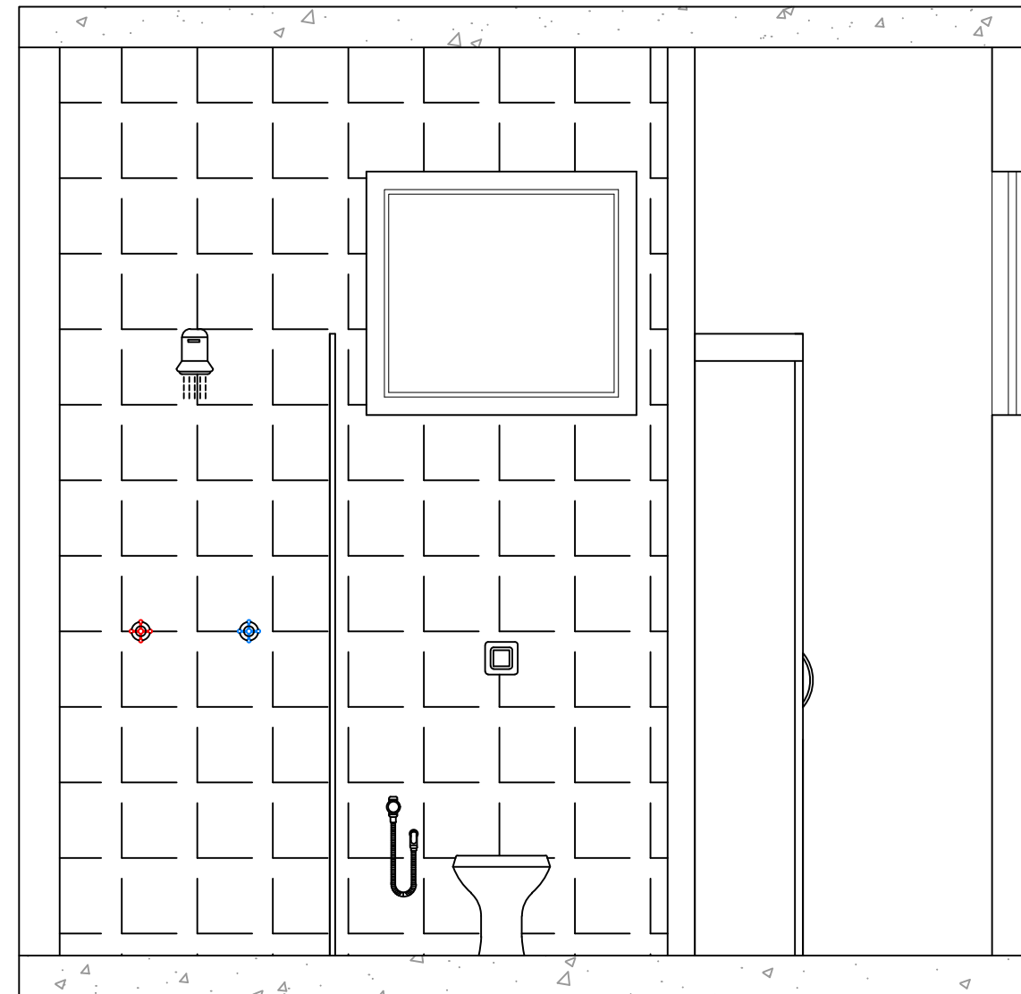
CORTE ESQUEMÁTICO ESCALA 1/25
