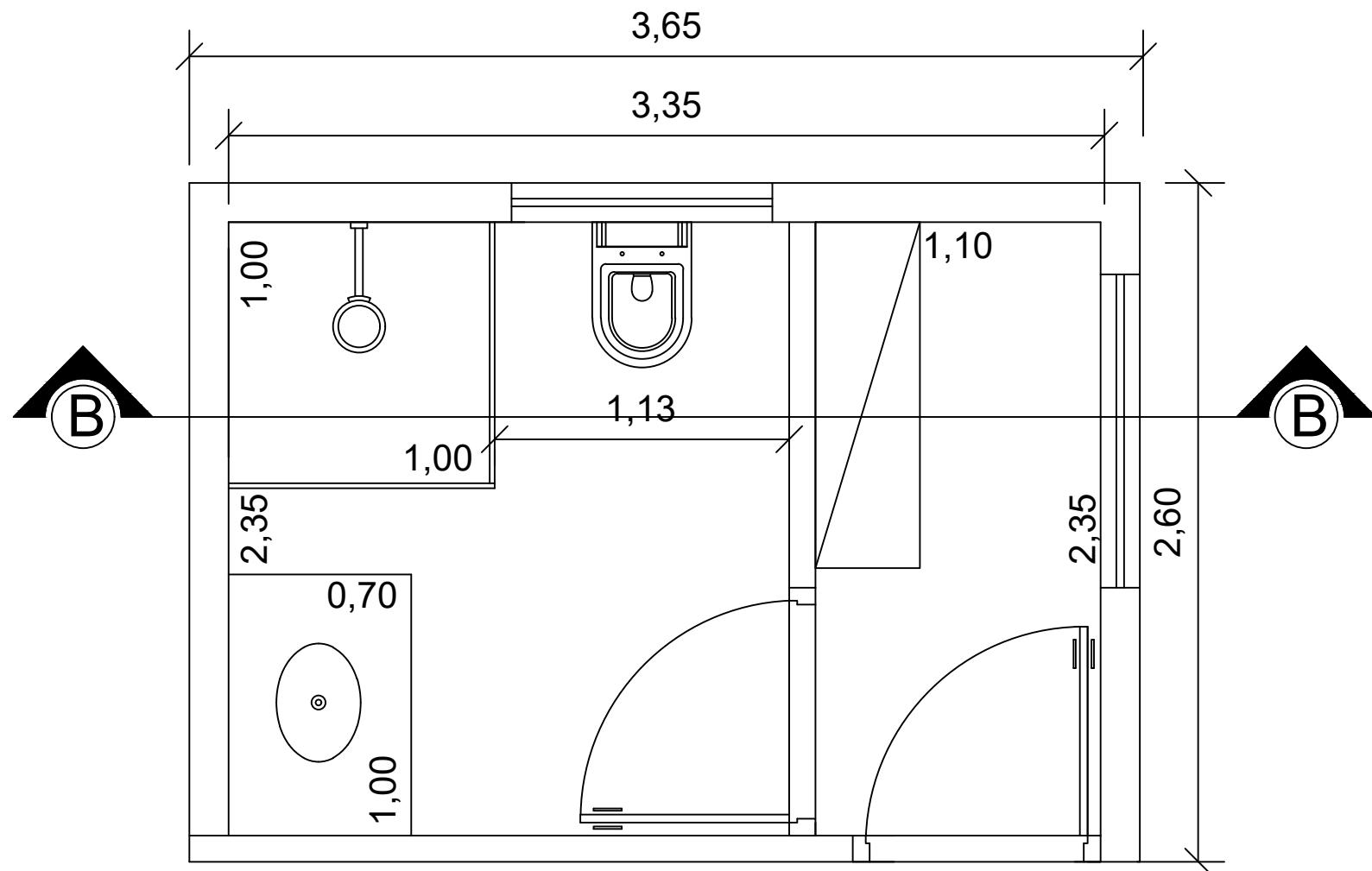
PLANTA DE LAYOUT ESCALA 1/25
