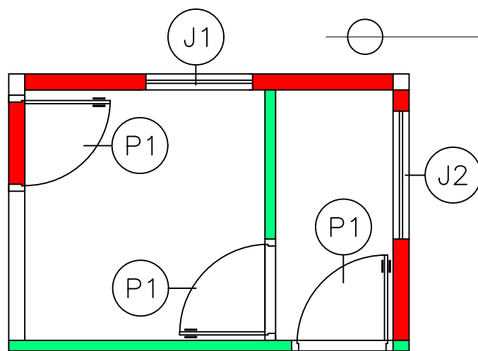
PLANTA DE DEMOLIÇÕES ESCALA 1/50
