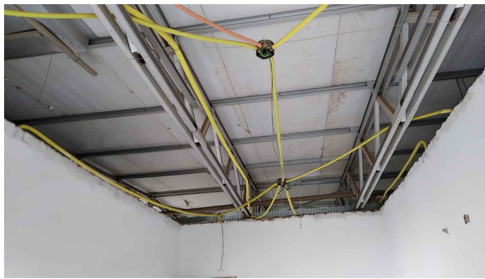
ELETRODUTOS PARA INSTALAÇÕES ELÉTRICAS DISTRIBUÍDOS
