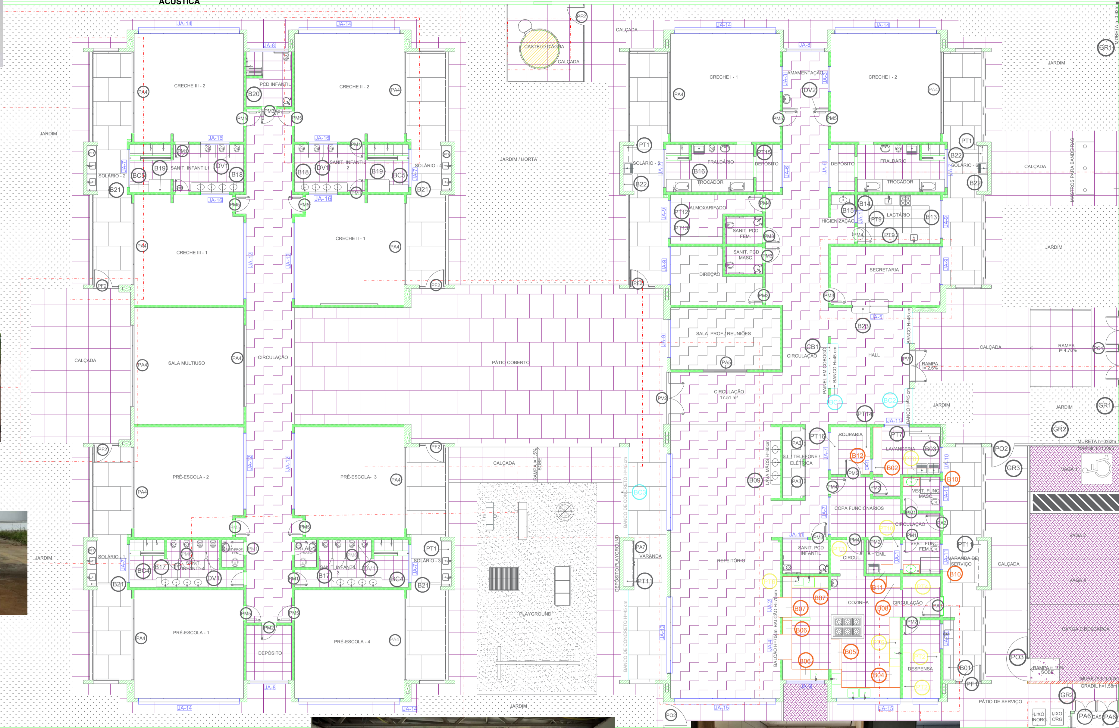
PLANTA BAIXA ESC: 1/125
