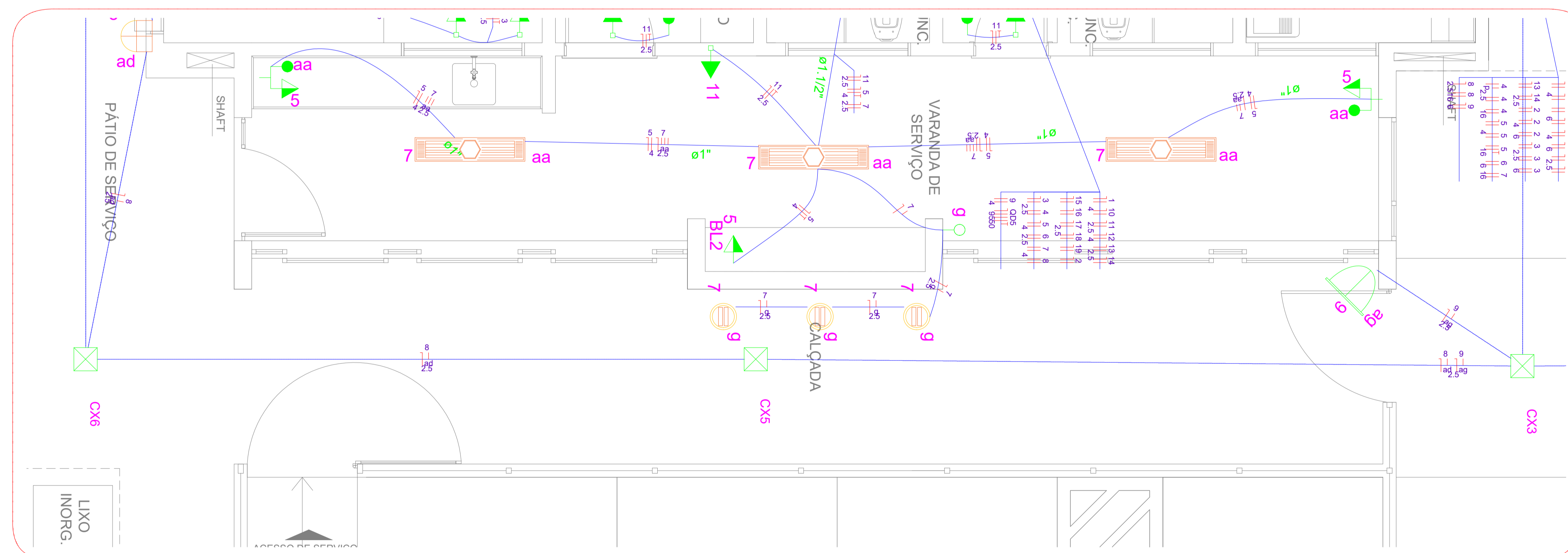
DISTRIBUIÇÃO DE REDE ELÉTRICA ESC: S/E
