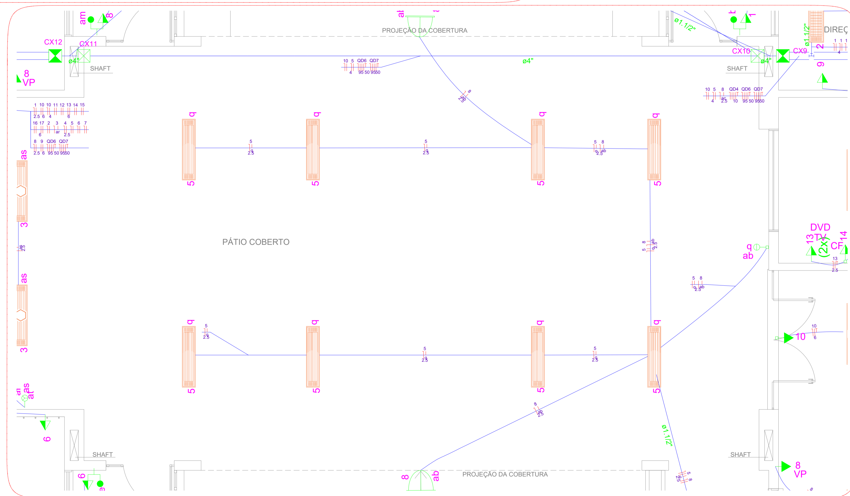
DISTRIBUIÇÃO DE REDE ELÉTRICA ESC: S/E
