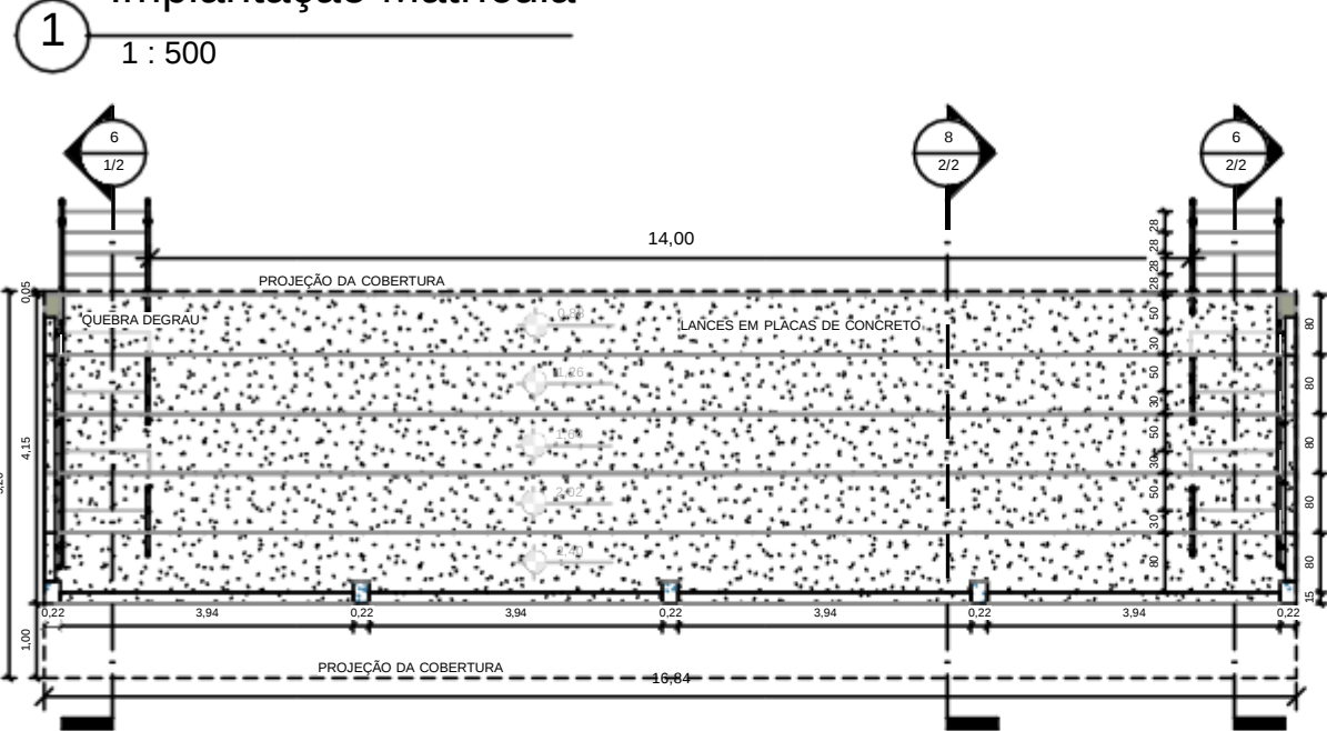
4 Planta Baixa 1 : 75
