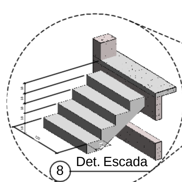
8 Det. Escada
