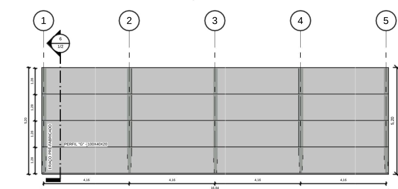
5 Cobertura 1 : 75
