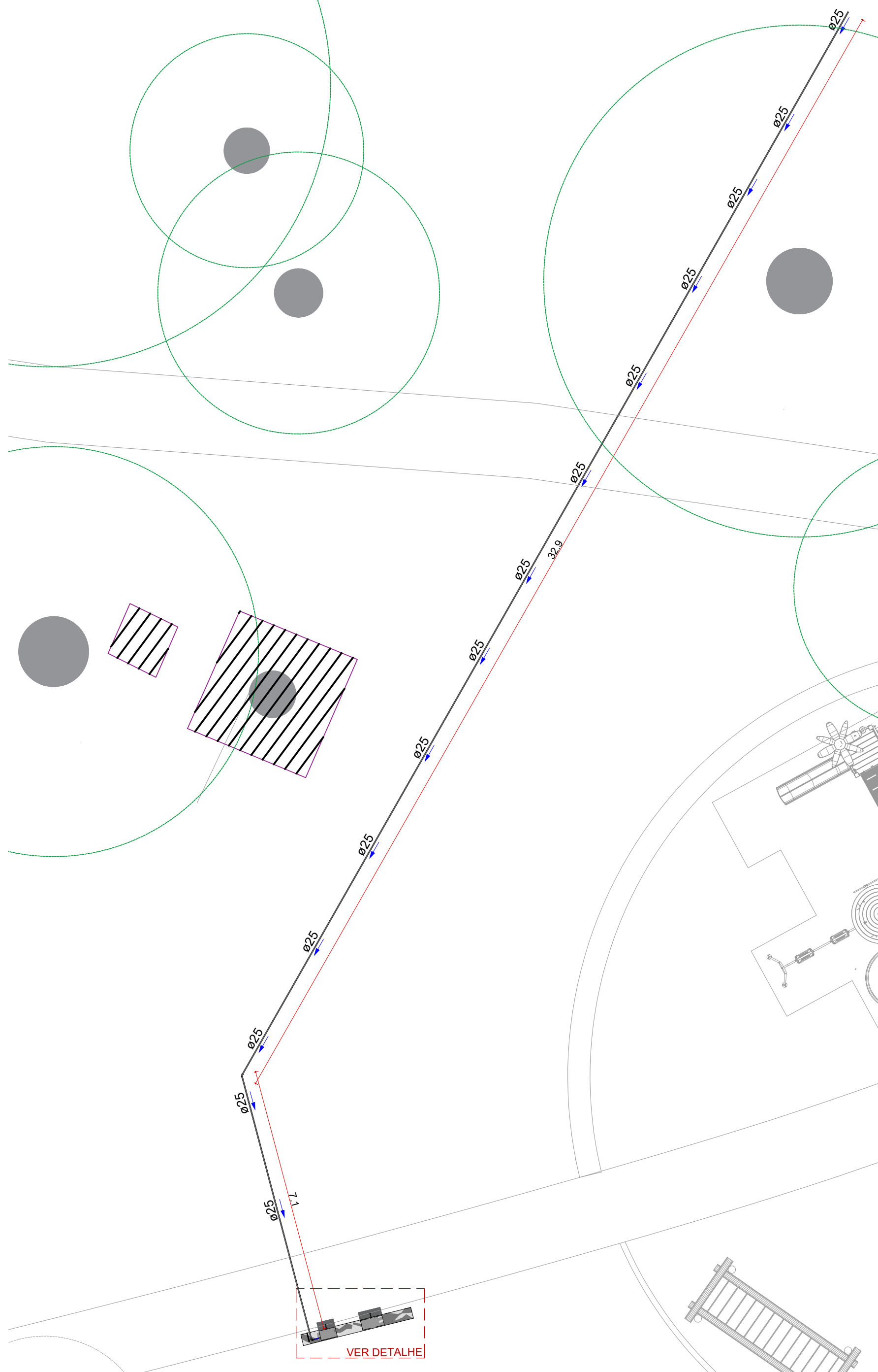
ÁGUA FRIA - BEBEDOURO Escala 1:100
