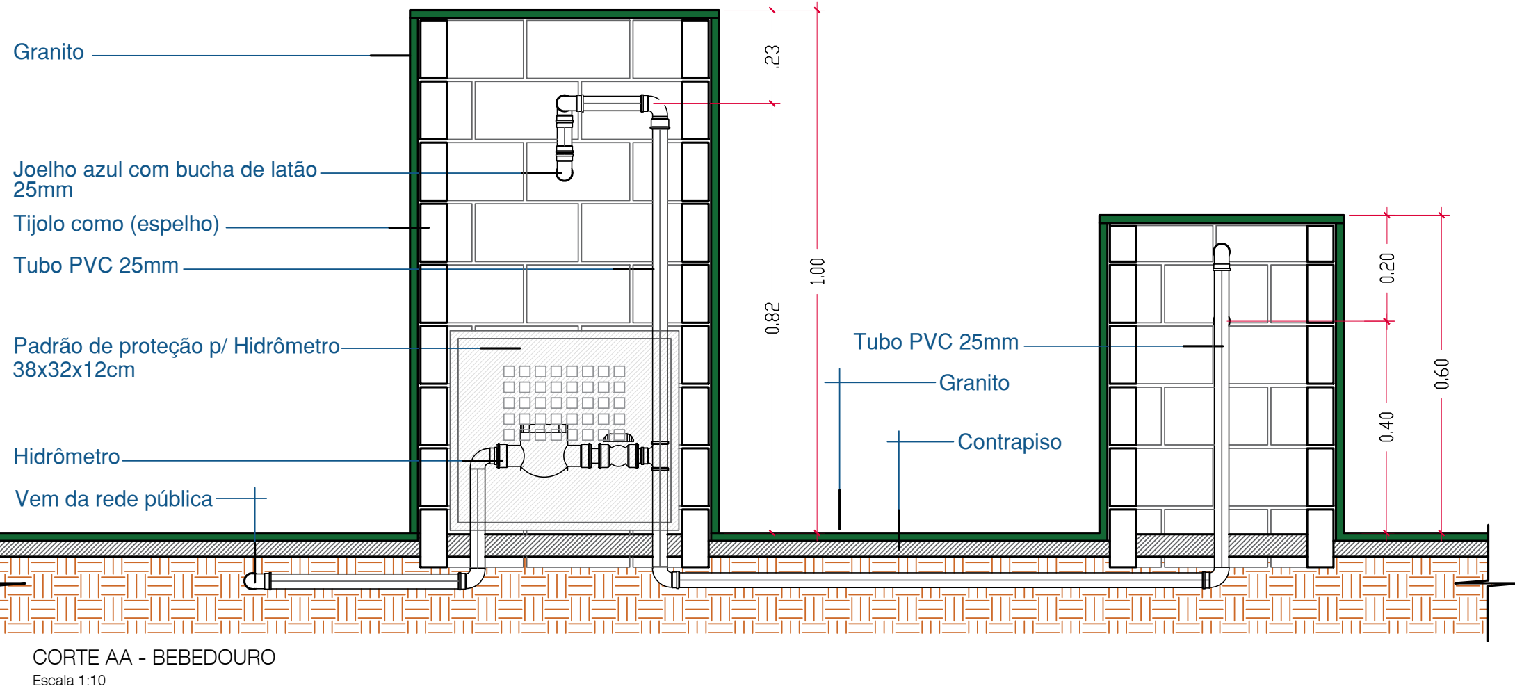
CORTE AA - BEBEDOURO Escala 1:10
