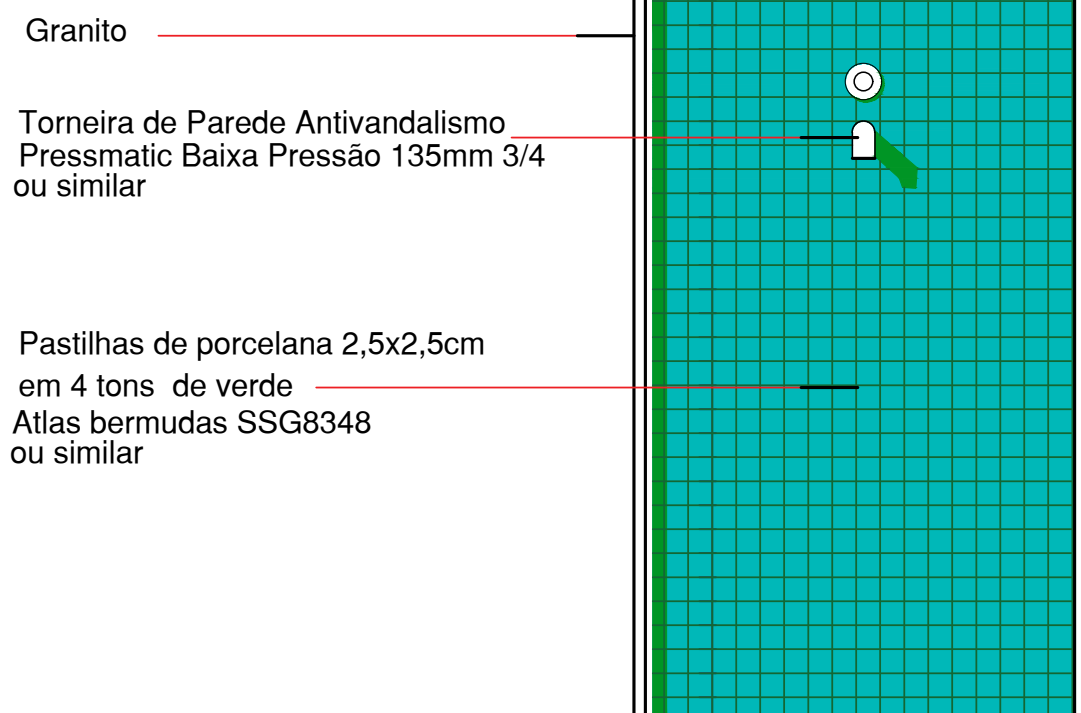
VISTA BEBEDOURO Escala 1:10
