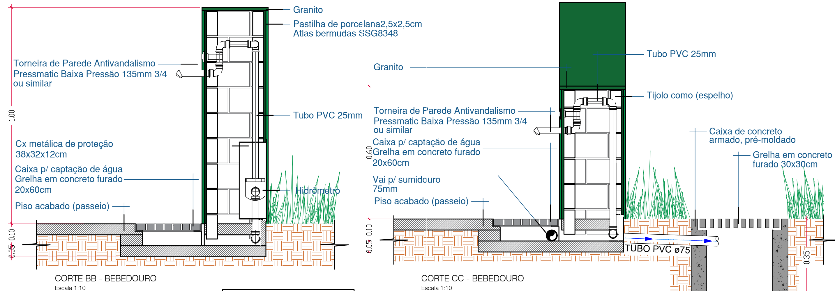
CORTE BB - BEBEDOURO Escala 1:10
