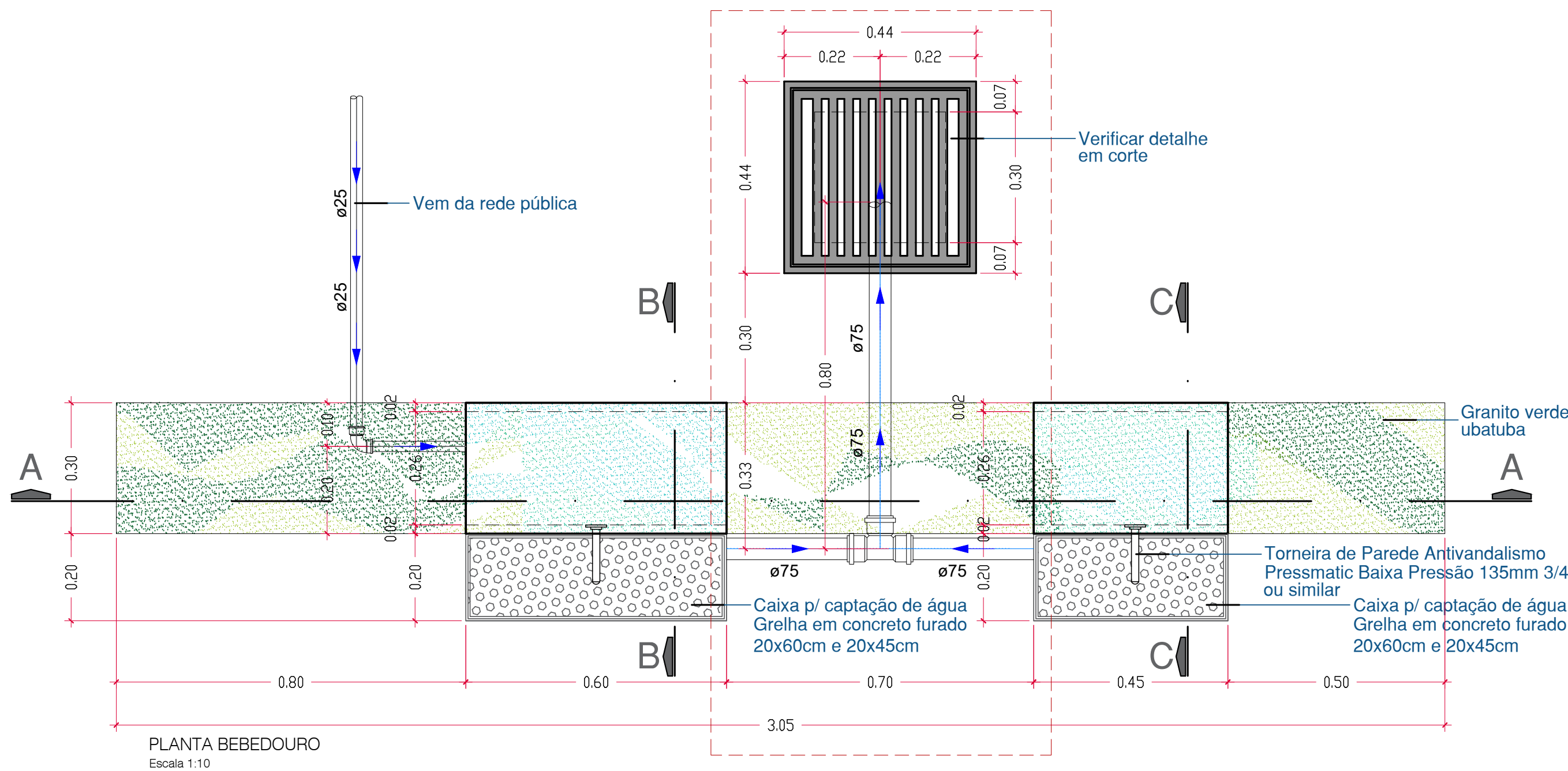
PLANTA BEBEDOURO Escala 1:10
