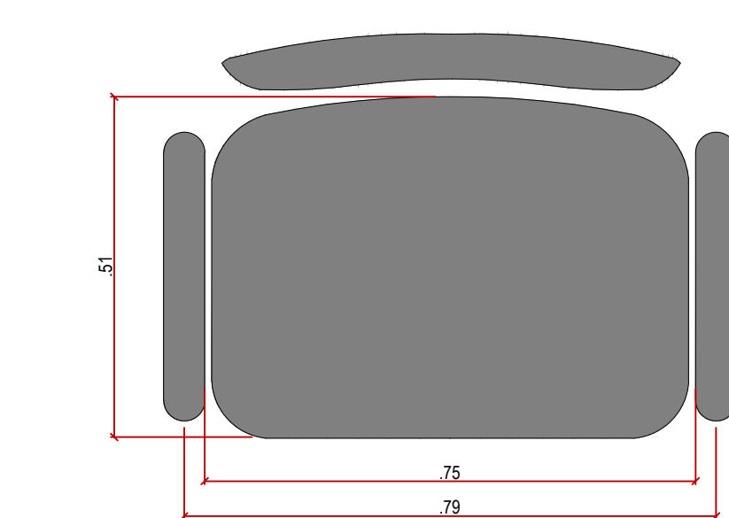
77 DETALHE 08 - assento para pessoas obesas
