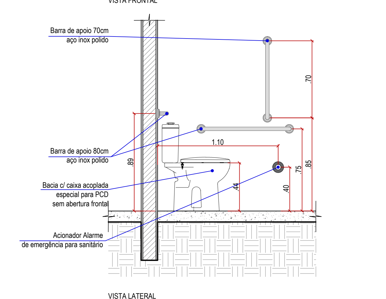
80 DETALHE 11 - Bacia sanitária PCD
