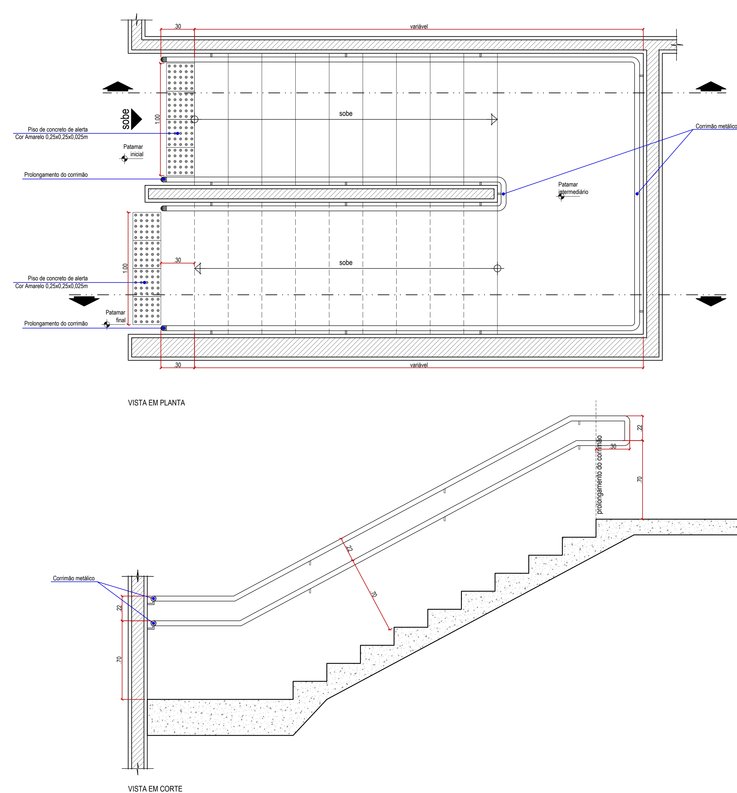
75 DETALHE 06 - Corrimão escadas
