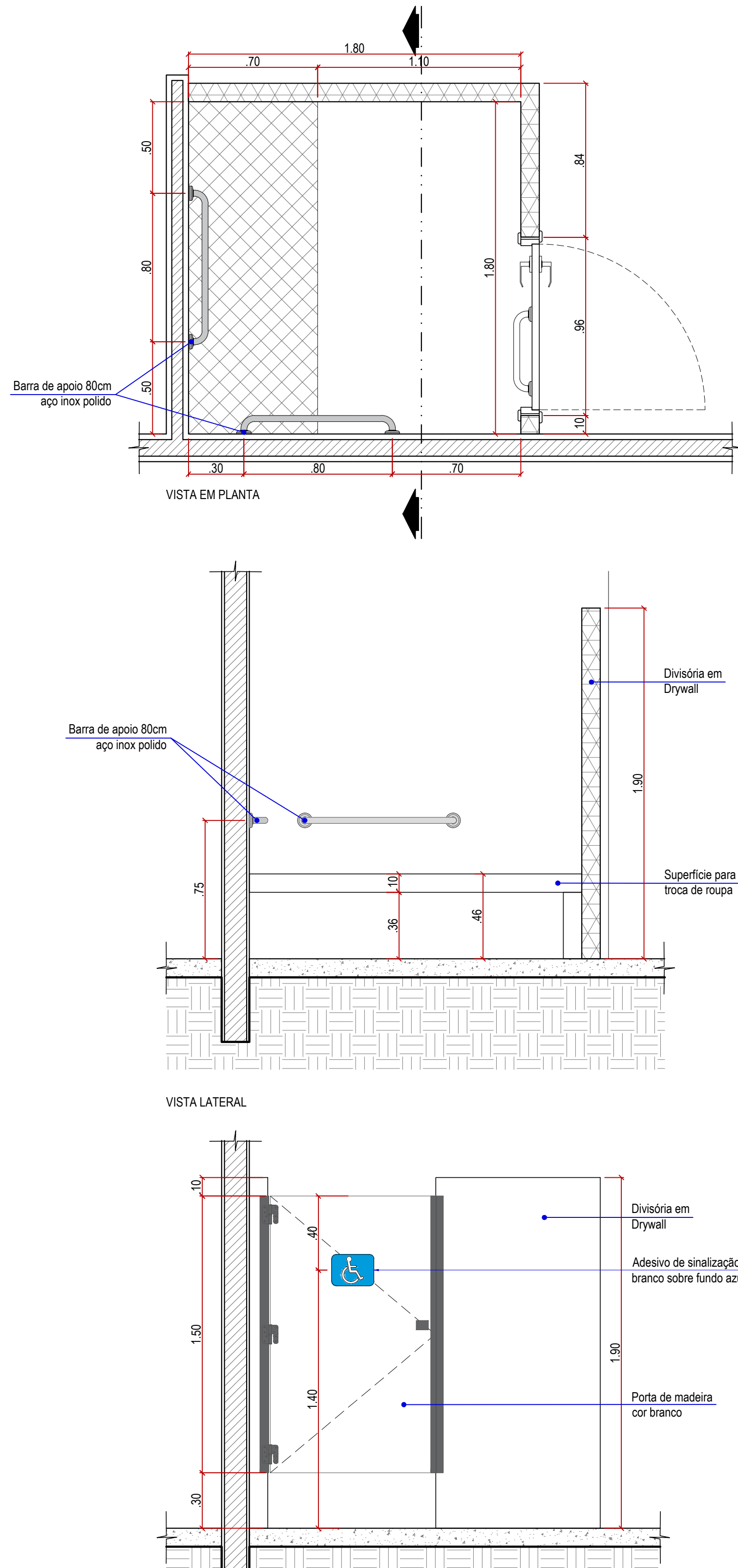
23 DETALHE 13 - vestiário PCD
