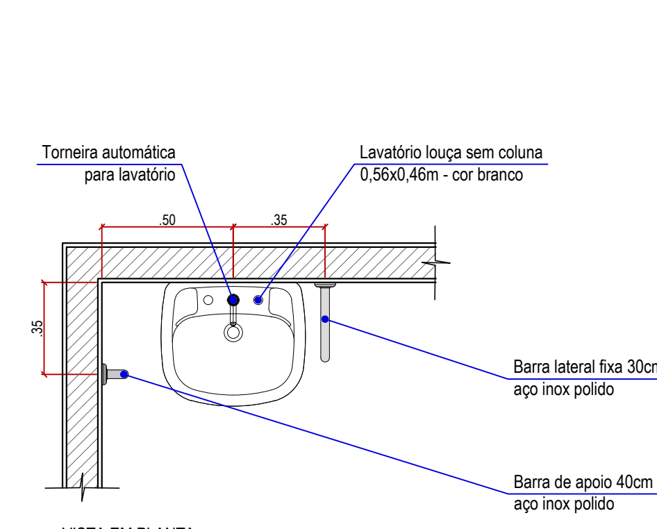
VISTA EM PLANTA
