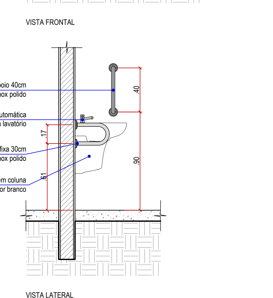
79 DETALHE 10 - Lavatório PCD
