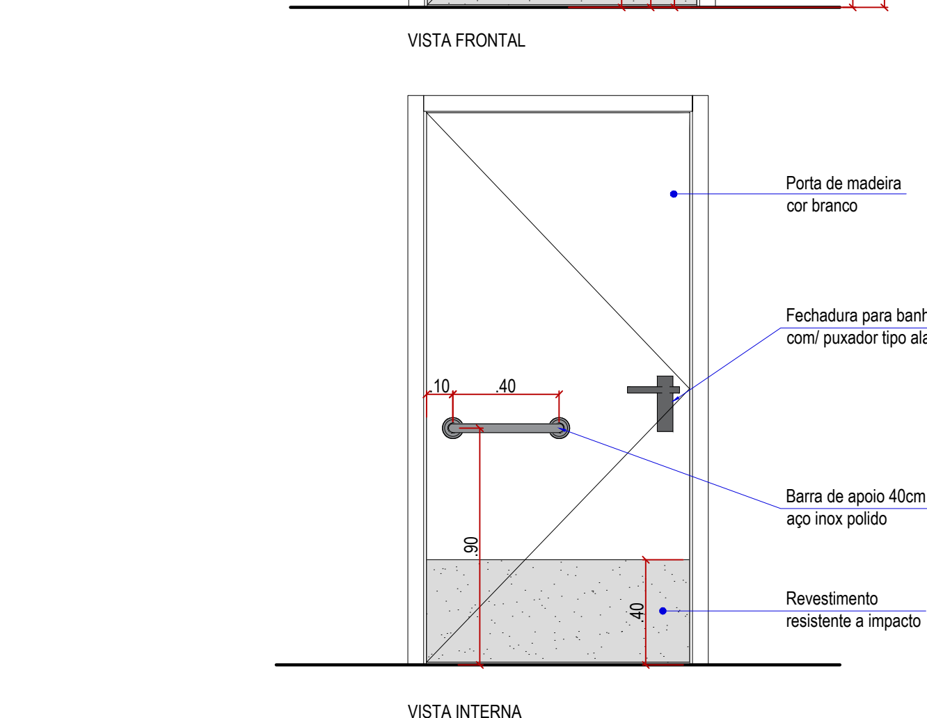
81 DETALHE 12 - Portas PCD (0,90x2,10m)
