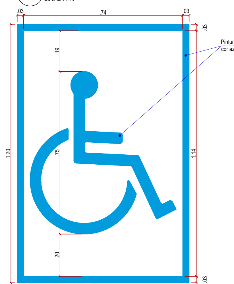
78 DETALHE 09 - espera P.C.R.
