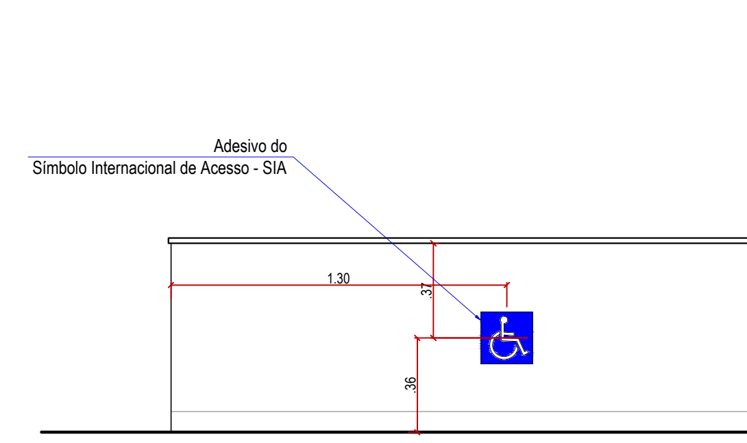
76 DETALHE 07 - sinalização balcões recepção / farmácia
