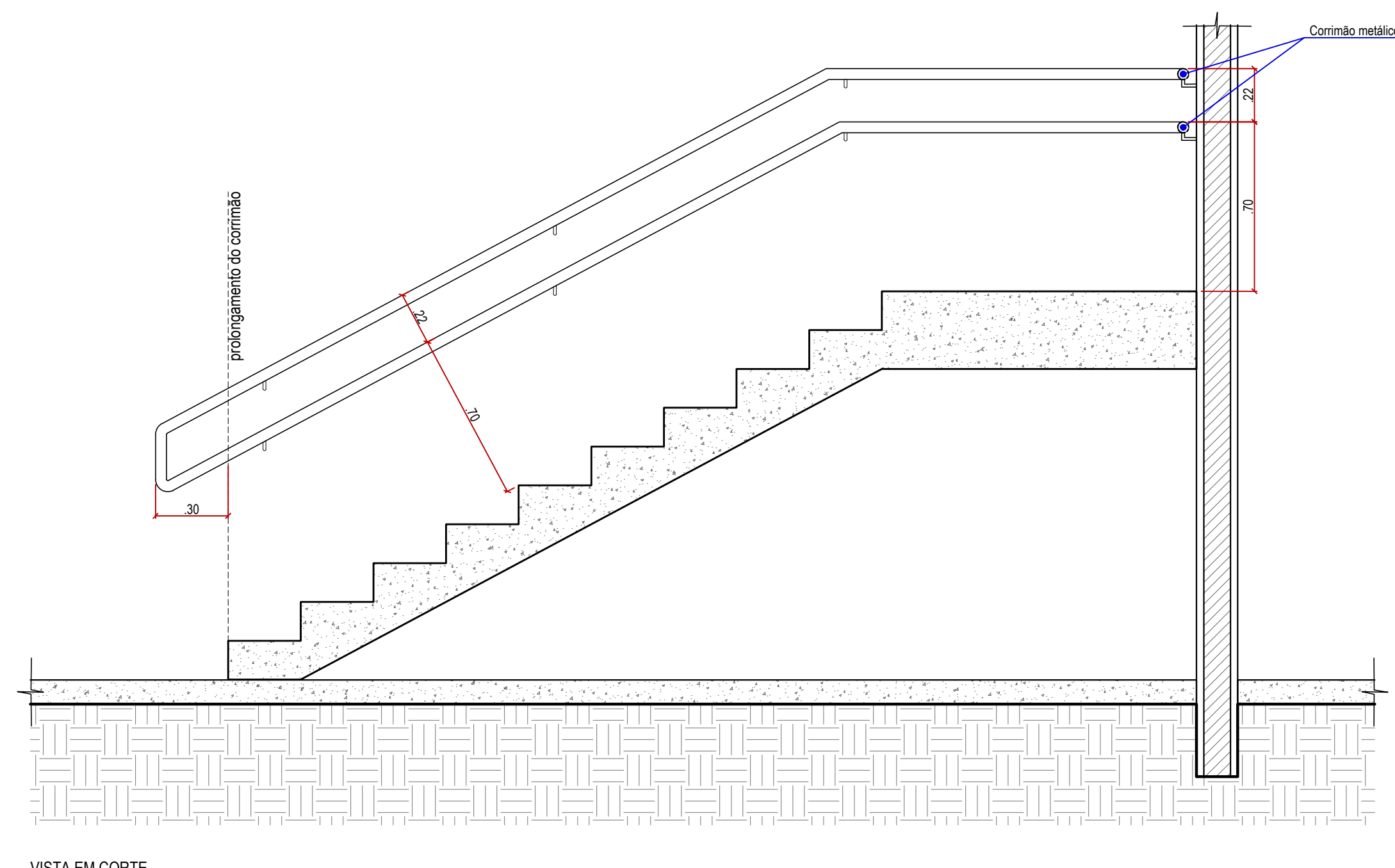
VISTA EM CORTE
