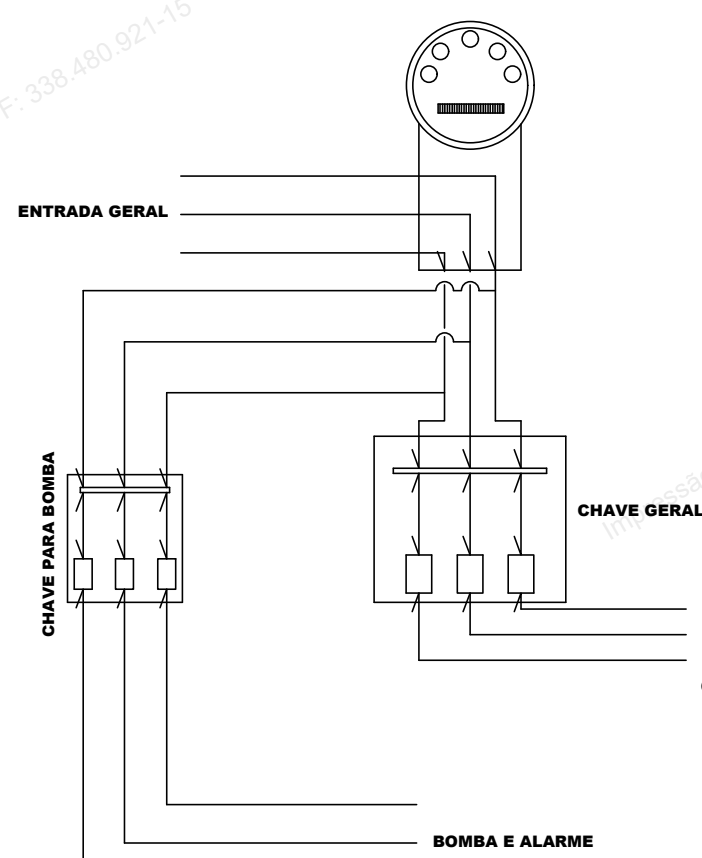
ESQUEMA DE LIGAÇÃO DA BOMBA E ALARME S/ESC.
