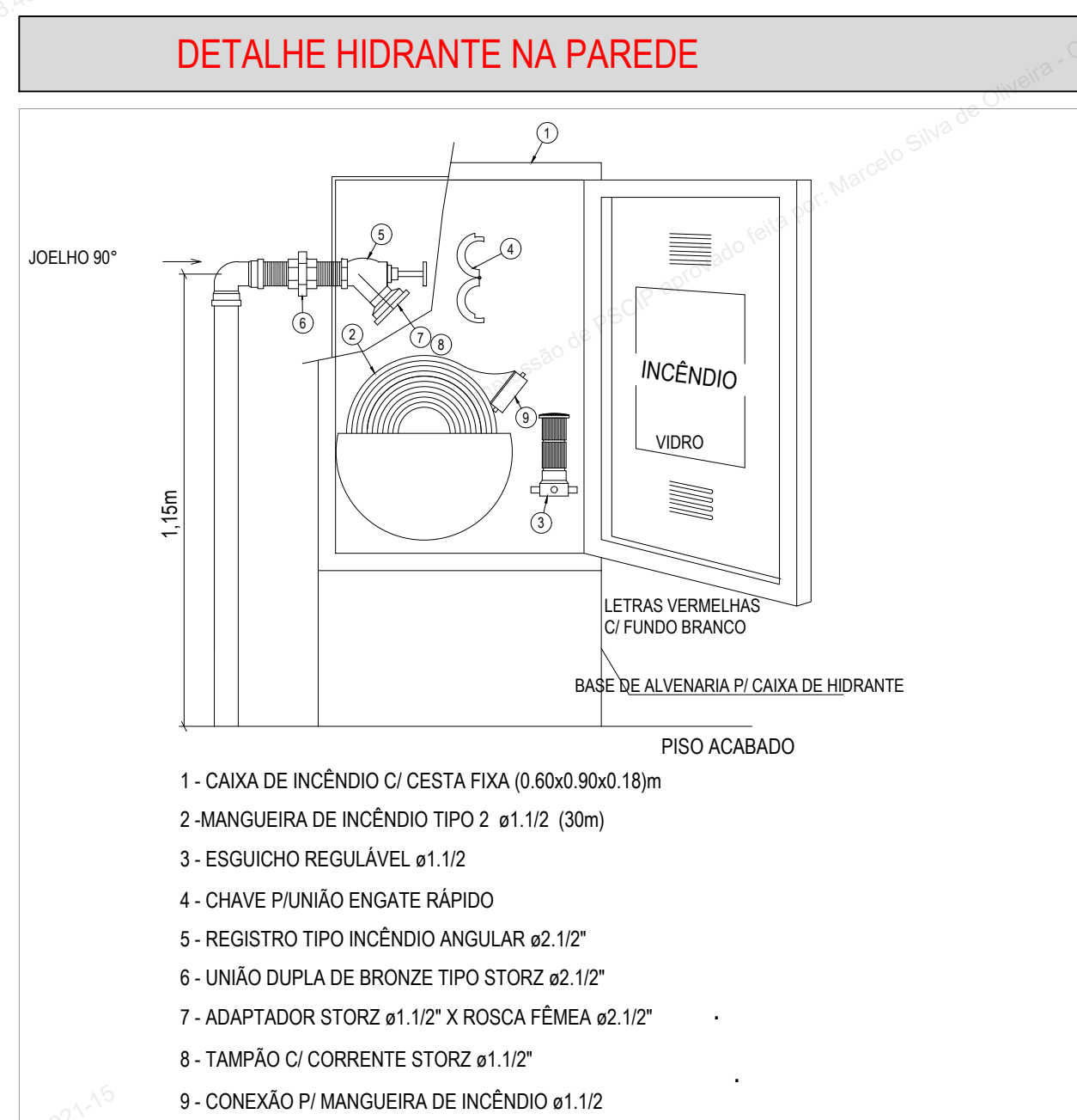
(DETALHE S/ ESCALA)
