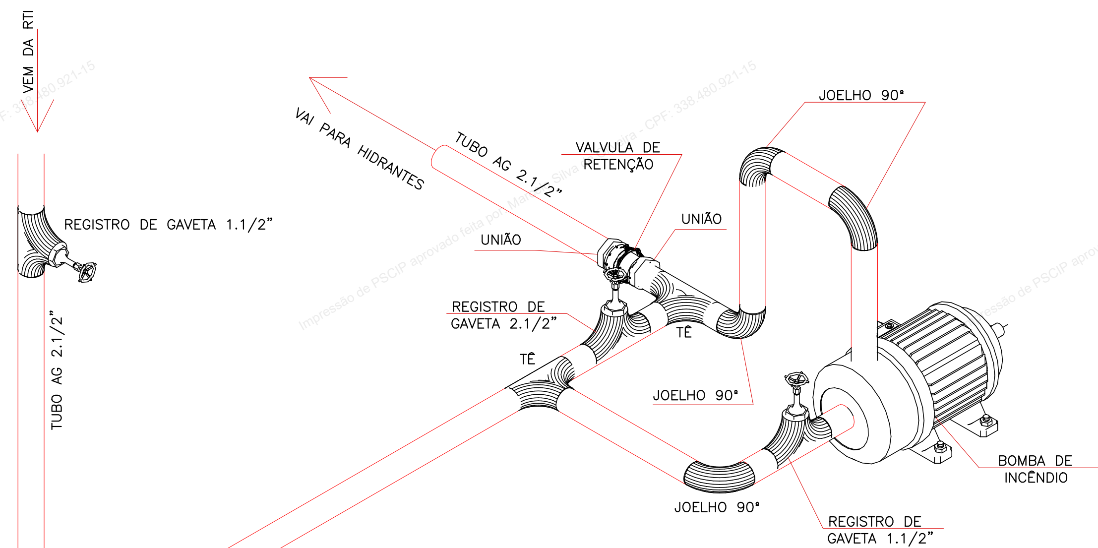
CONJUNTO MOTOR BOMBA CENTRIFUGA SCHNEIDER POT. 7,5CV TRIFASICO BPI-22 R/F 2 1/2" (ROTOR 155 mm) ou similar Hman: 42,00 mca Q=20,80 m3/h
