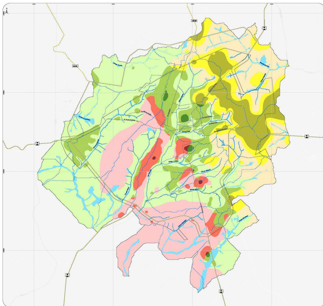
Figura 12 – Carta Geotécnica de Campo Grande
