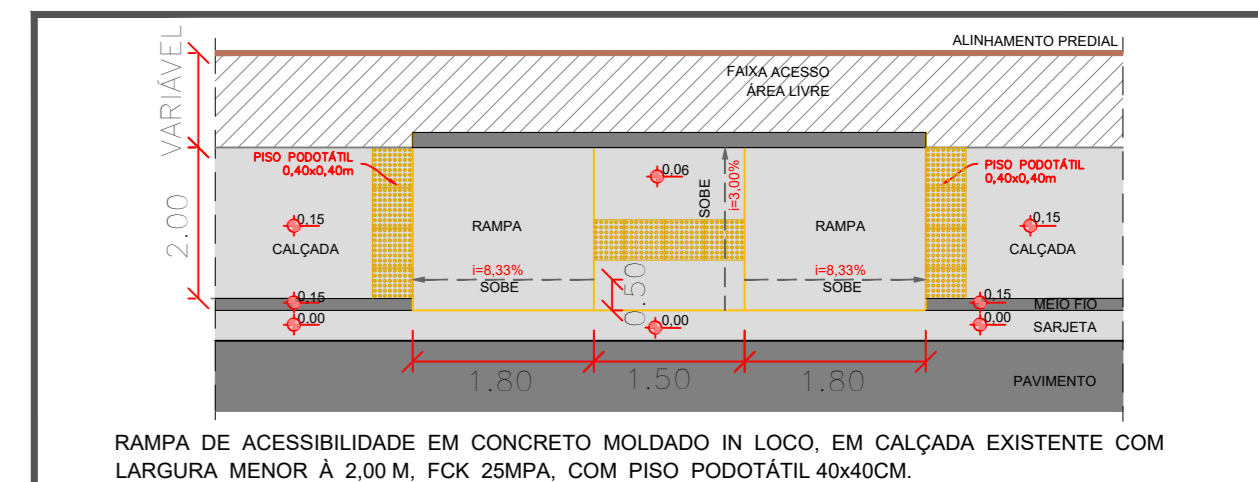
ESC.: 1/75
