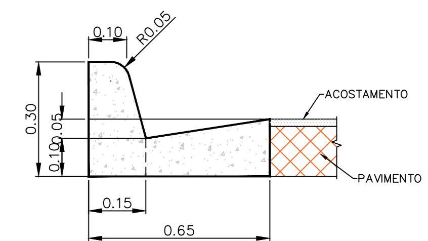
MFC01 ESC=1:10
