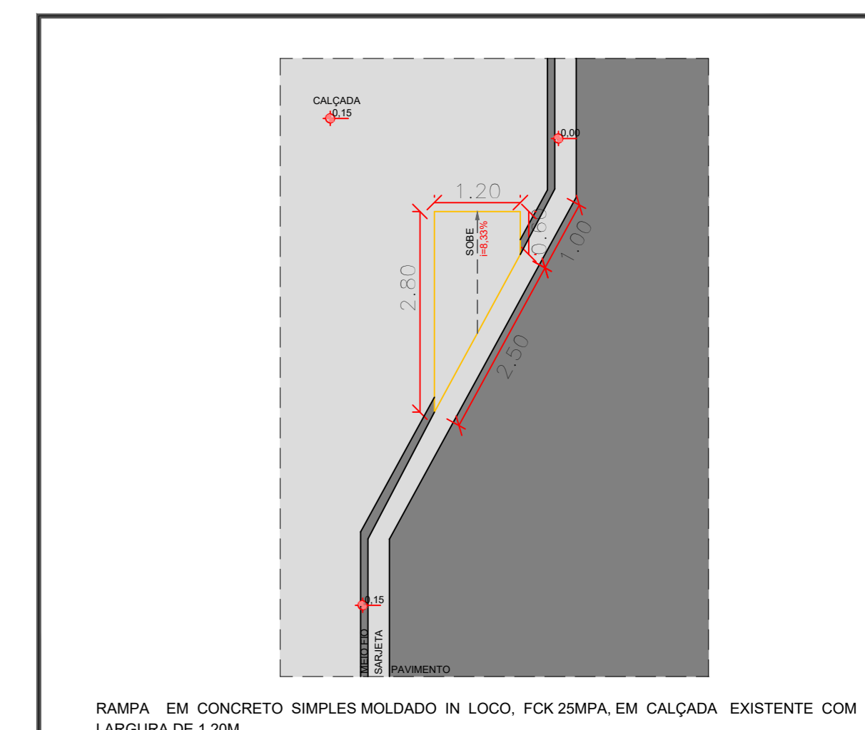
RAMPA EM CONCRETO SIMPLES MOLDADO IN LOCO, FOX 20MPA, EM CALÇADA EXISTENTE COM LARGURA DE 1,20M. ESC.: 1/75
