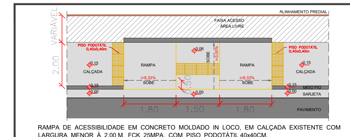
RAMPA DE ACESSIBILIDADE EM CONCRETO MOLDADO IN LOCO, EM CALÇADA EXISTENTE COM LARGURA MENOR A 2,00 M. FOX 20MPA, COM PISO PODOTÁTIL 40x40CM. ESC.: 1/75
