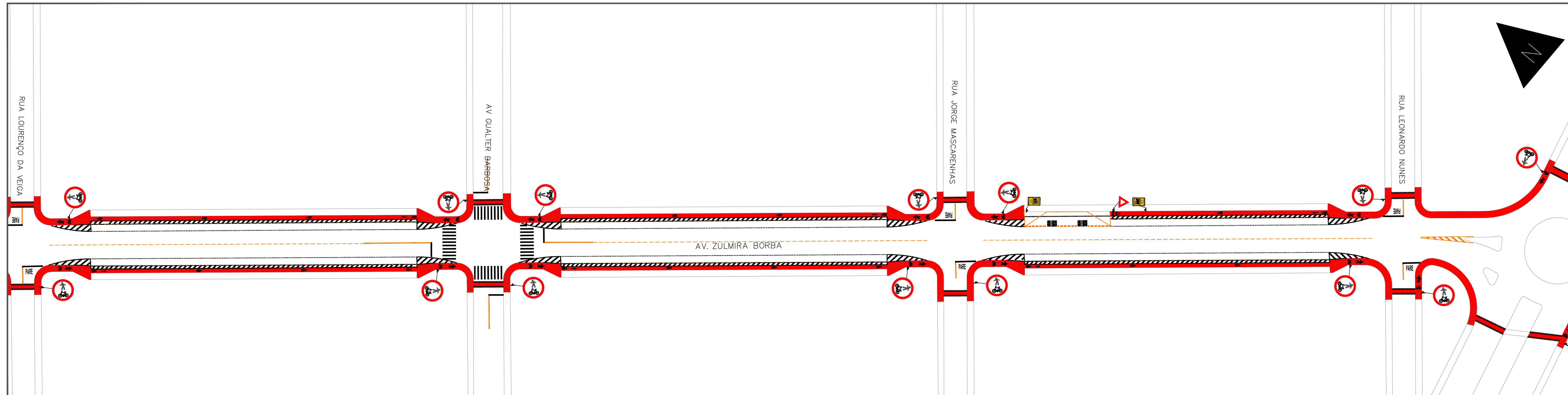
4 - PLANTA DE SINALIZAÇÃO ESC.: 1/500
