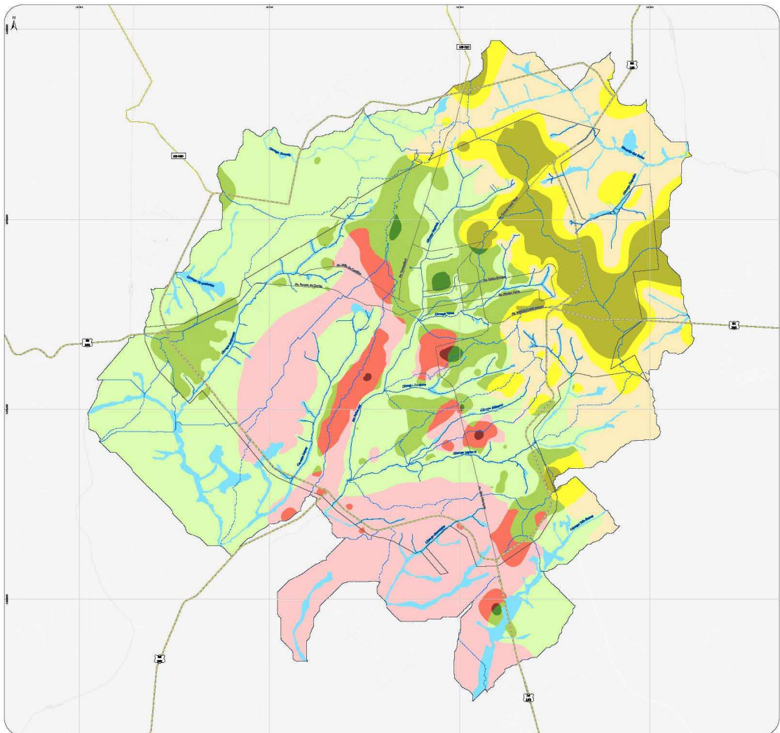
Figura 12 – Carta Geotécnica de Campo Grande
