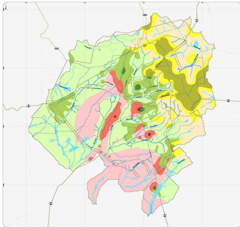
Figura 16 – Carta Geotécnica de Campo Grande
