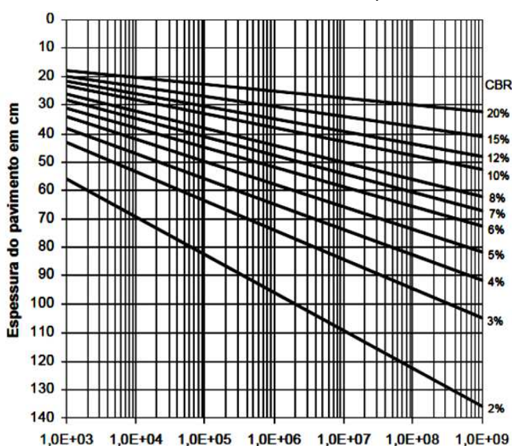
Figura 18 – Ábaco de dimensionamento de pavimentos flexíveis
