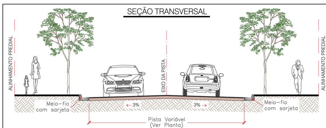
Figura 17 – Seção Transversal Tipo - Pavimentação
