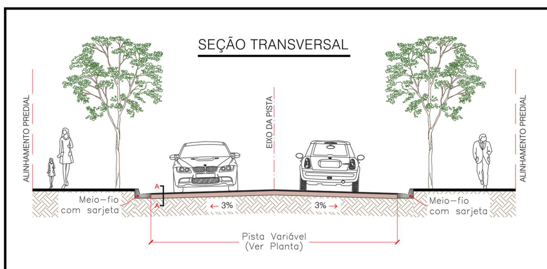
Figura 17 – Seção Transversal Tipo - Pavimentação
