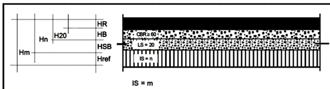
Figura 14 – Coeficiente estrutural “K” para cada tipo de base
