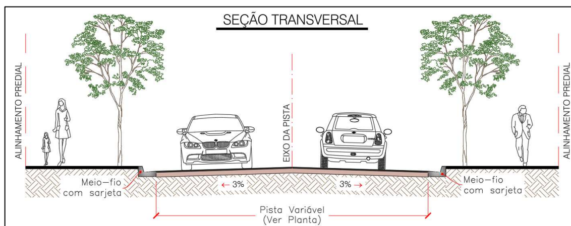
Figura 11 – Seção Transversal Tipo - Pavimentação
