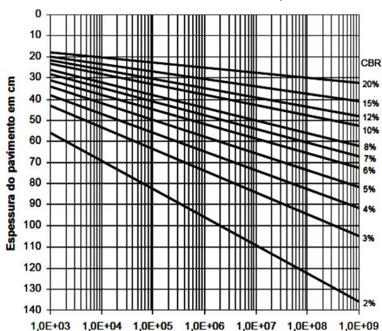
Figura 12 – Ábaco de dimensionamento de pavimentos flexíveis
