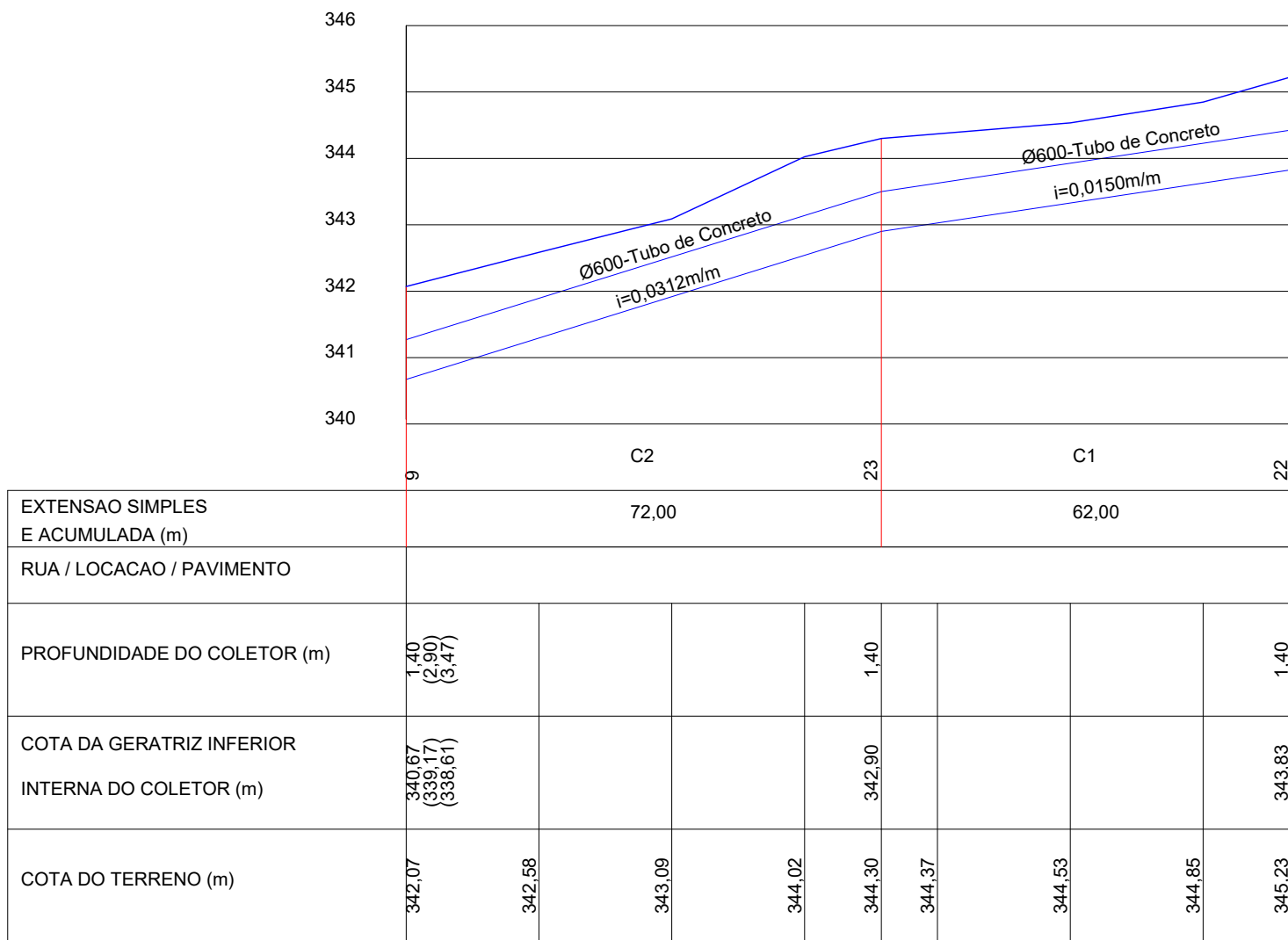
02 PERFIL DA REDE Esc.: 1:1000
