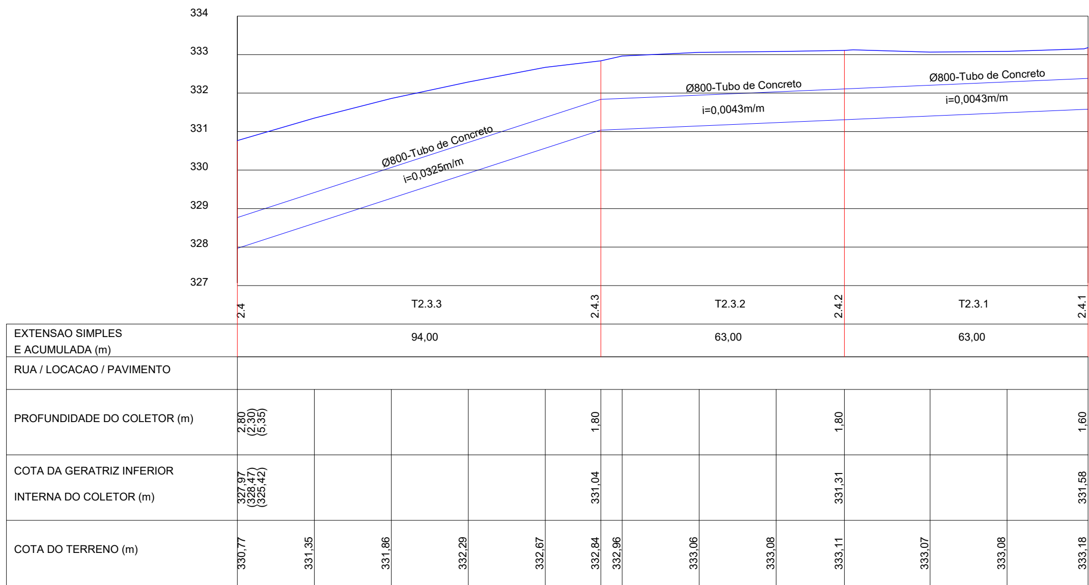
02 PERFIL DA REDE Esc.: 1:1000
