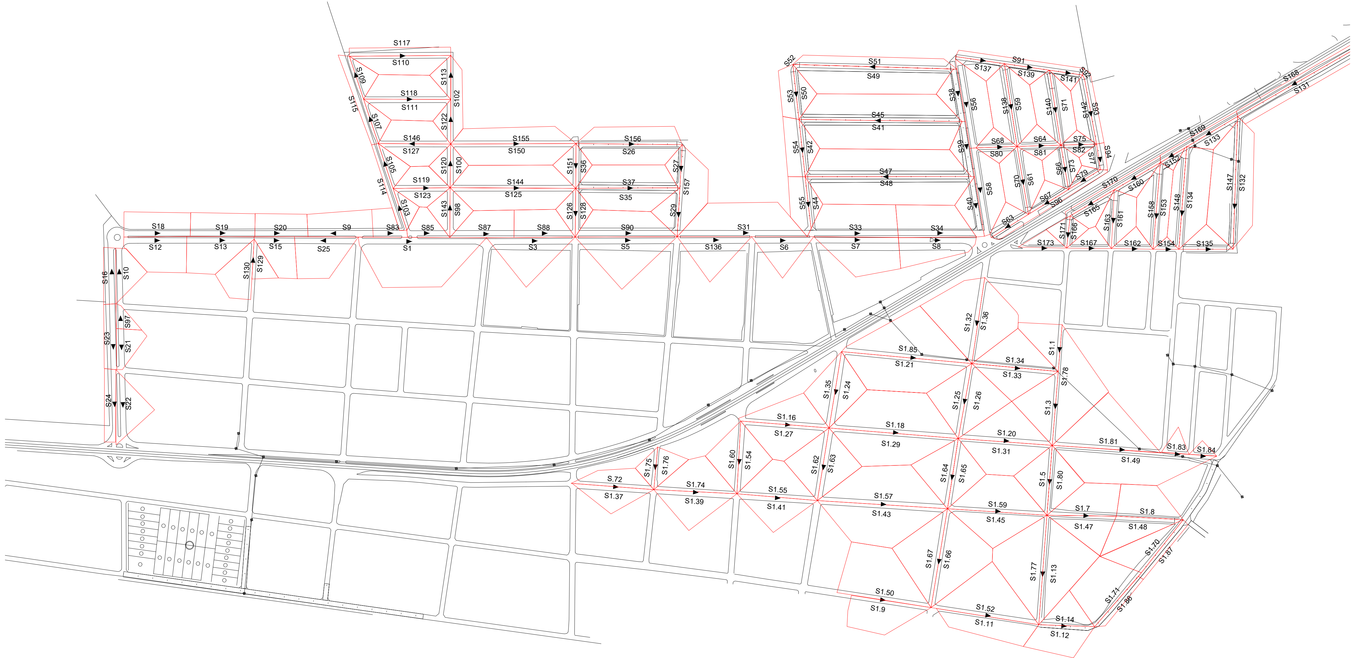
01 PLANTA BAIXA - REDE DE DRENAGEM Esc.: 1:2000
