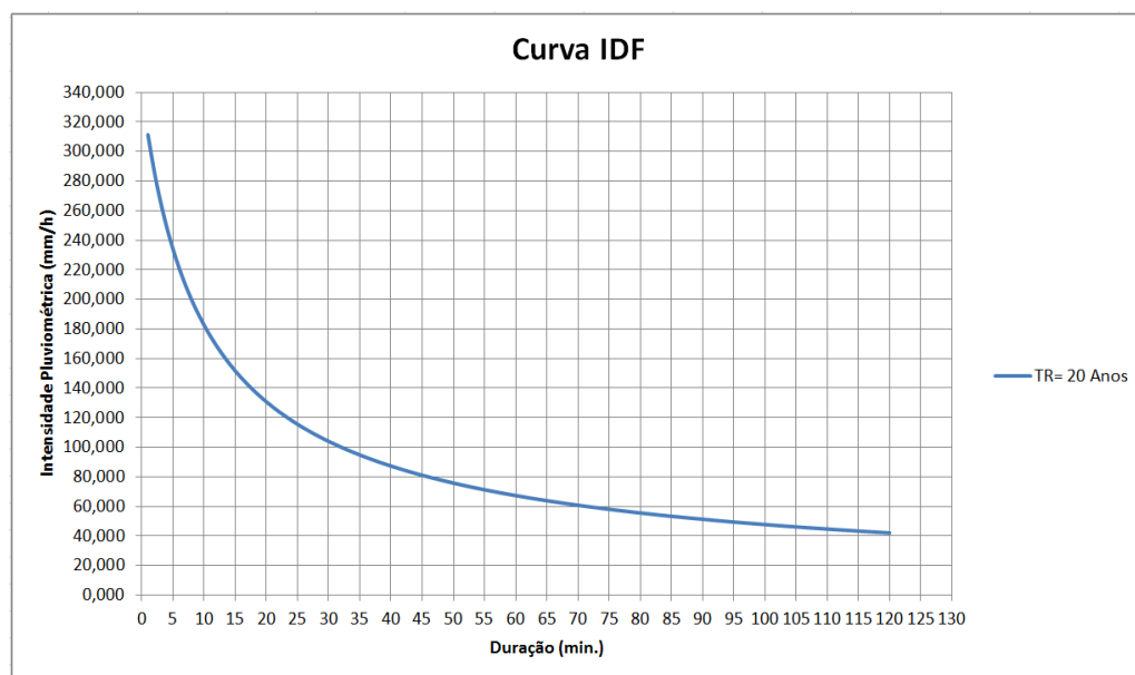
Figura 2 – Curva IDF para TR= 20 anos.
