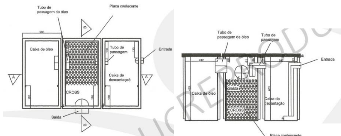
Figura 1 - Planta baixa e corte SAO - Cross Mallton do Brasil
