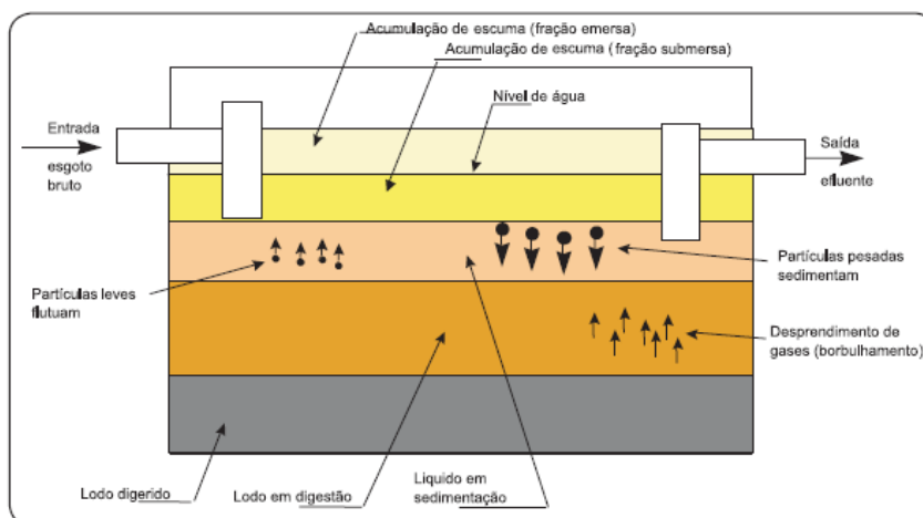
Figura 7 - Funcionamento de um tanque séptico (Adaptado de FUNASA, 2007)
