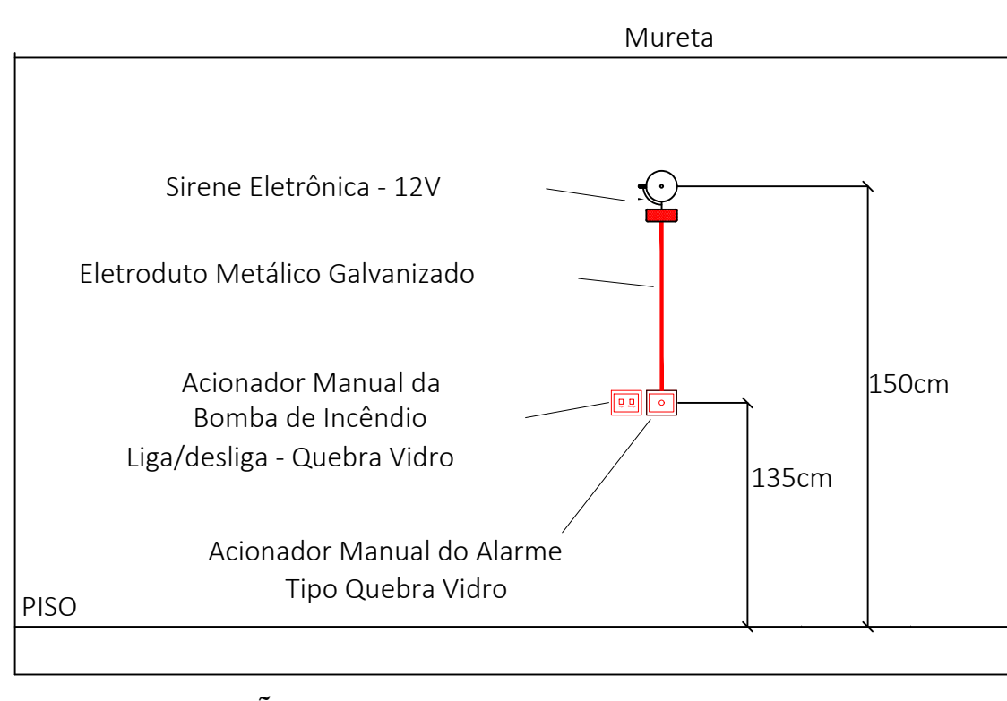
INSTALAÇÃO DO ACIONADOR MANUAL DO ALARME, DA SIRENE E DA BOTOEIRA DE INCÊNDIO
