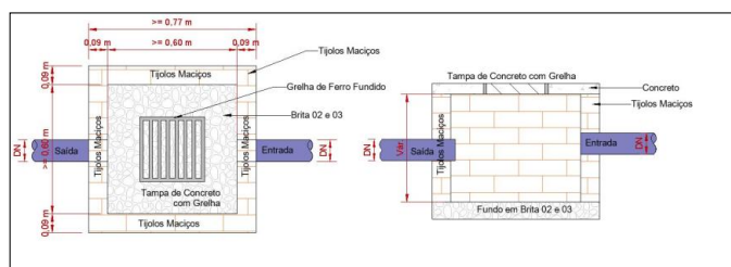
Figura: Caixa de areia em alvenaria
