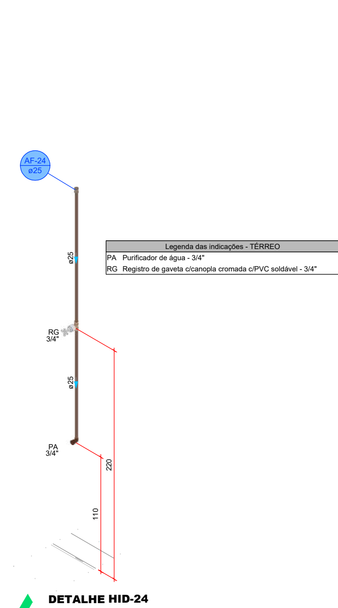
DETALHE HID-24 1:25
