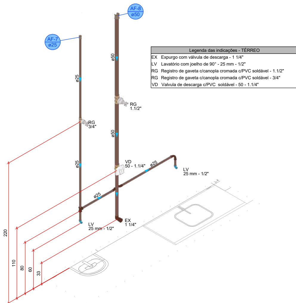
DETALHE HID-8 1:25
