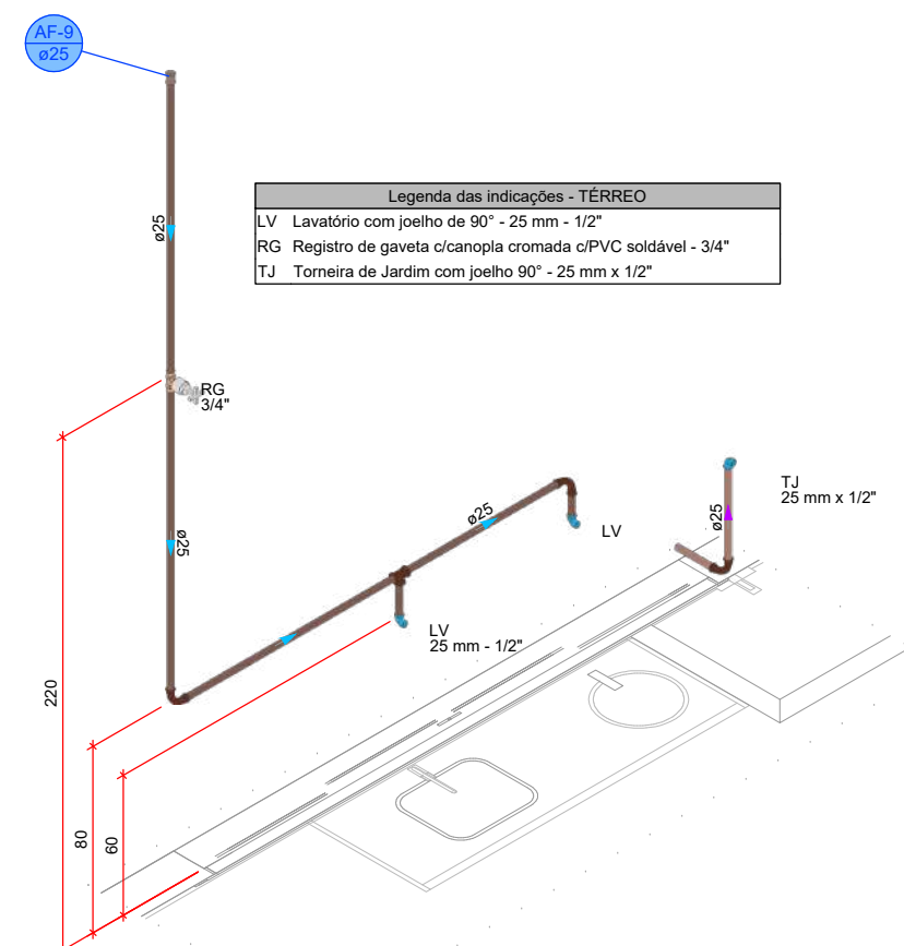
DETALHE HID-11 1:25
