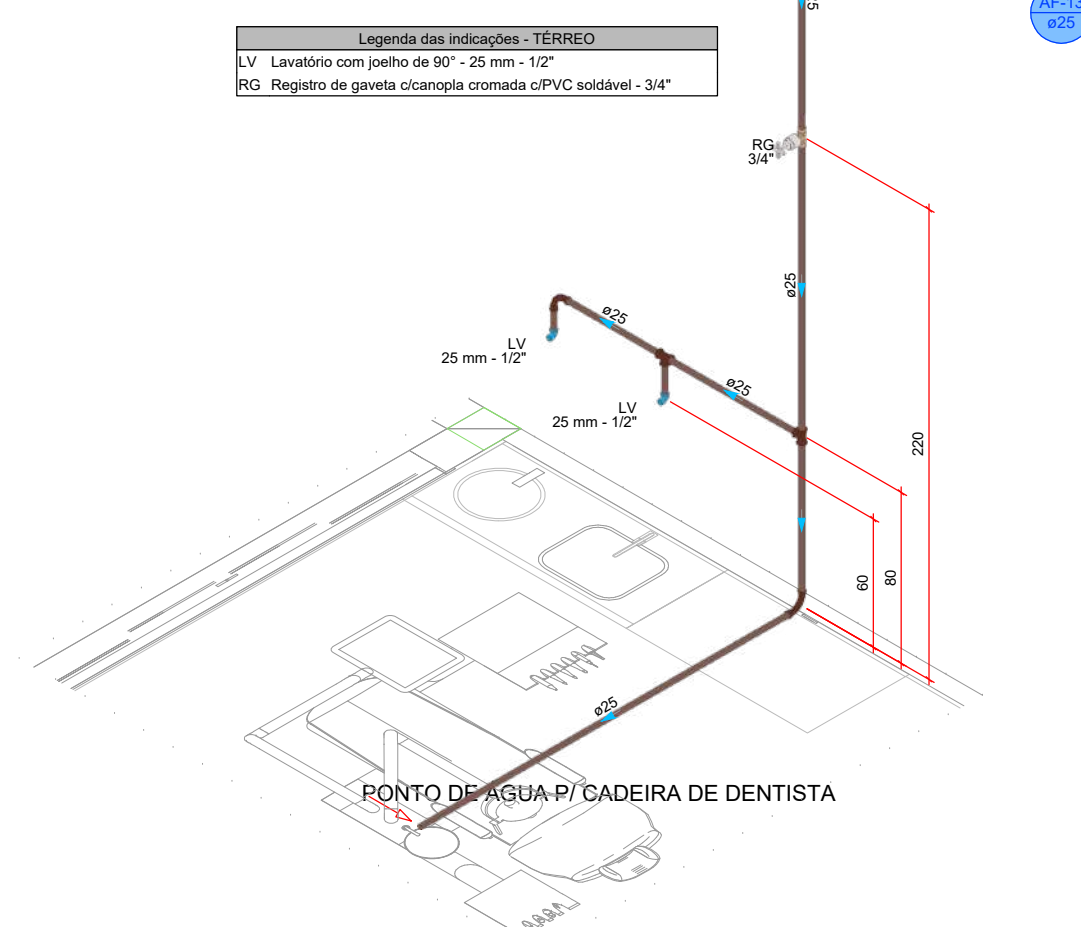
DETALHE HID-13 1:25
