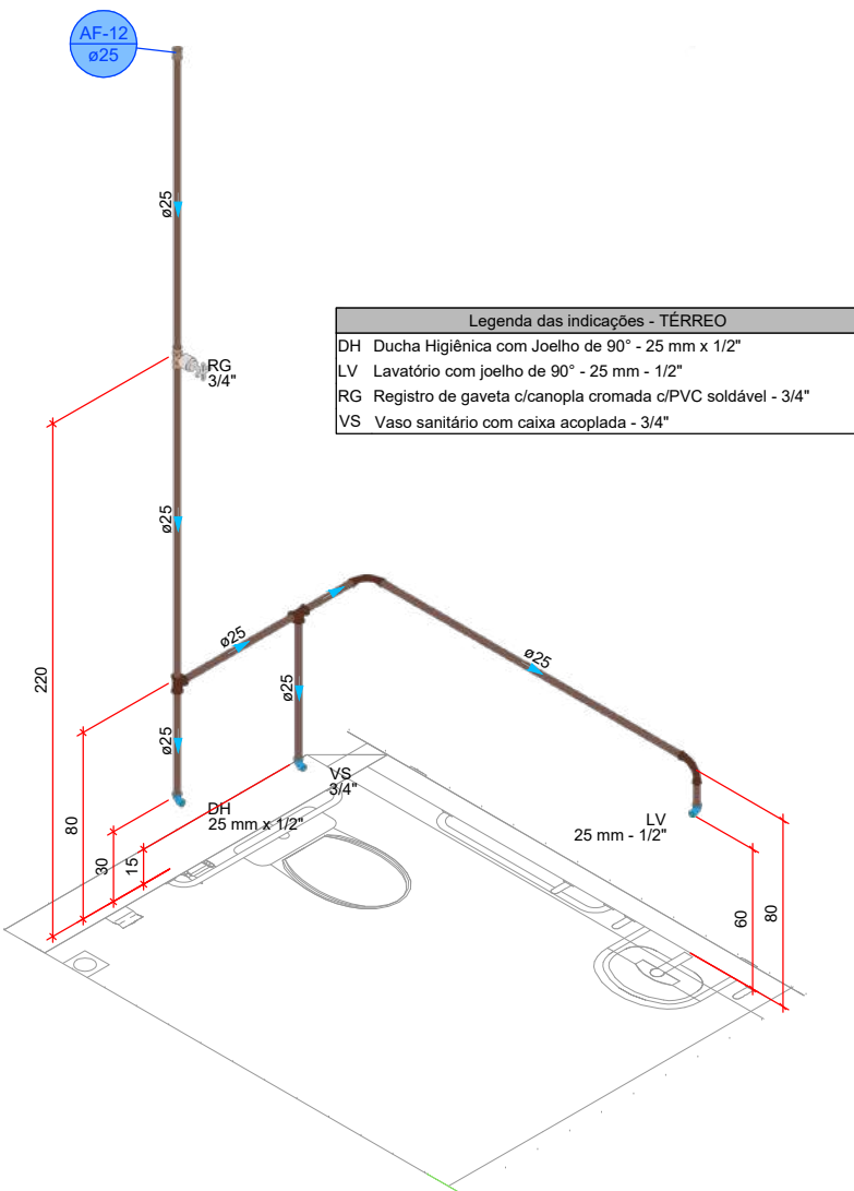
DETALHE HID-12 1:25
