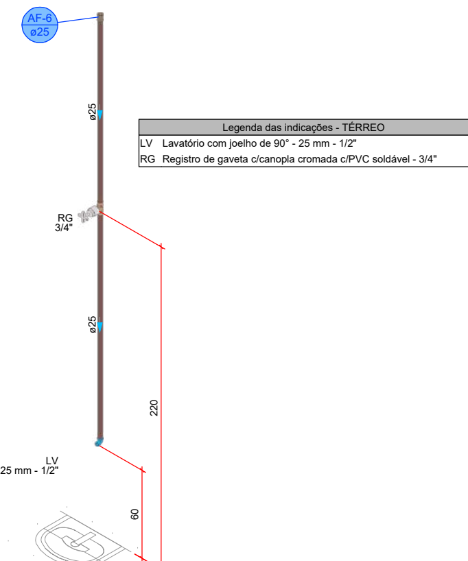
DETALHE HID-7 1:25
