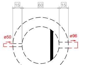
Caixa de gordura - TÉRREO Planta baixa - ESC. 1:25
