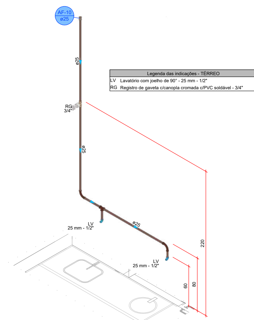
DETALHE HID-10 1:25
