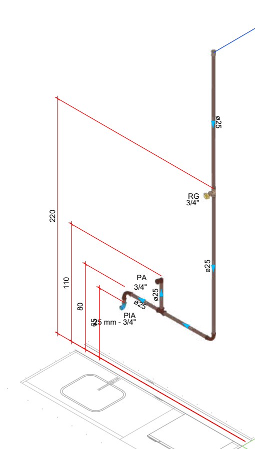
DETALHE HID-3 1:25
