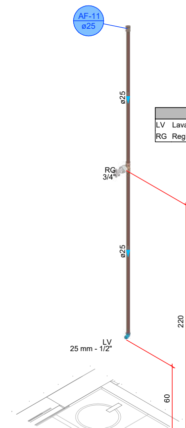
DETALHE HID-9 1:25
