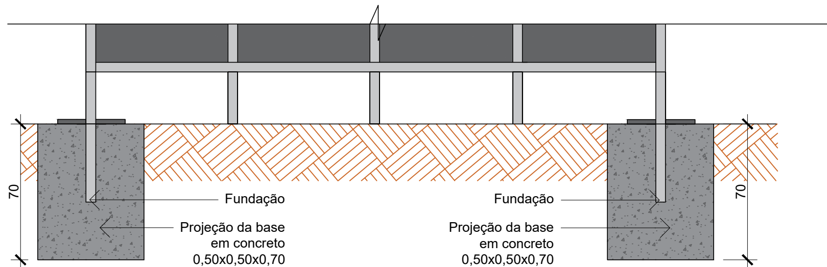
CORTE BB' FRONTAL - DET. FUNDAÇÃO ESC: 1/20
