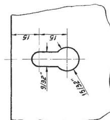
Detalhe do furo de sustentação da caixa d'água esc. 1:1
