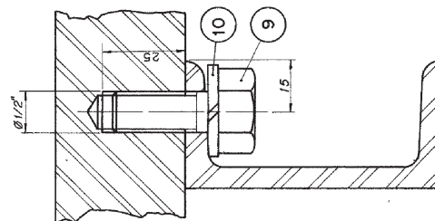
Detalhe da secção A
