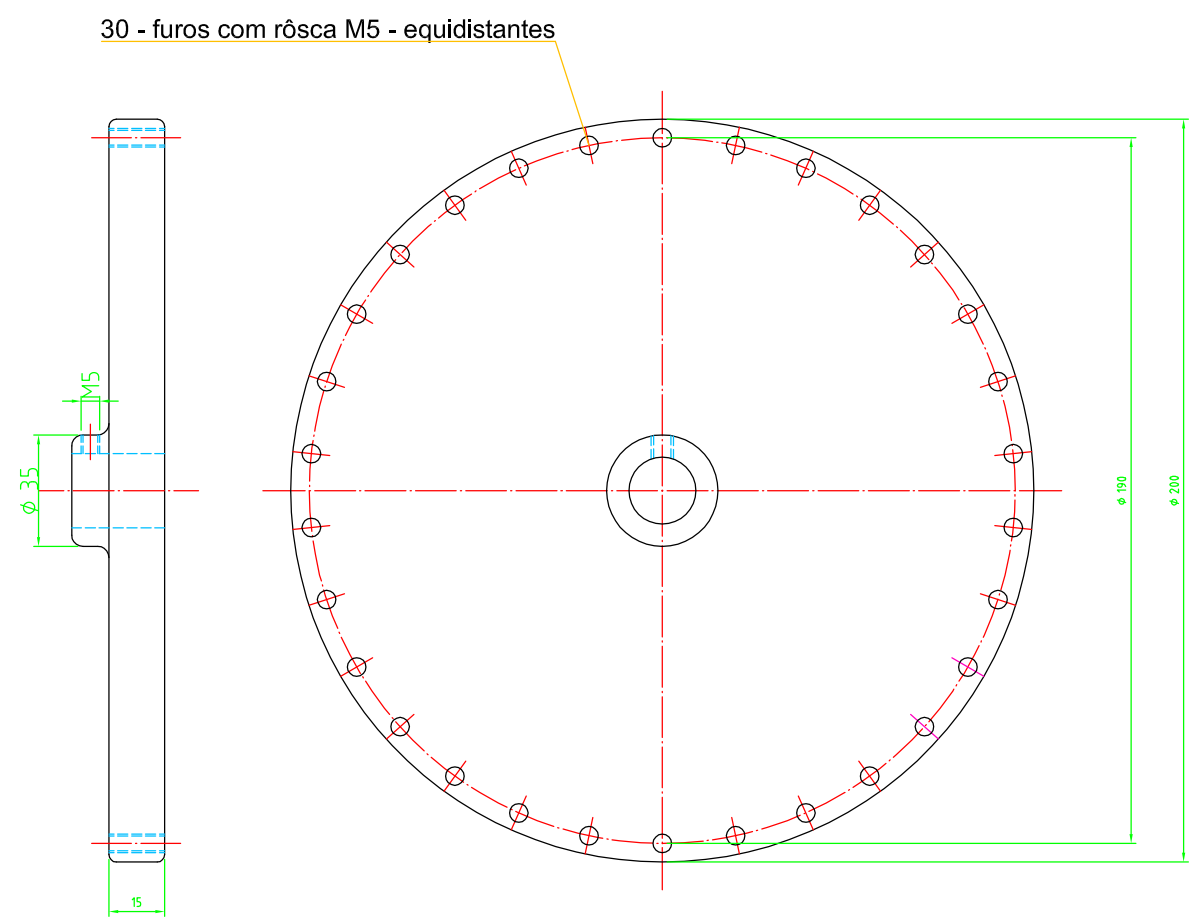
06 - Detalhe do disco para balanceamento Deve acompanhar 30 parafusos c/cab. sext int. M5x12 ou 15mm
