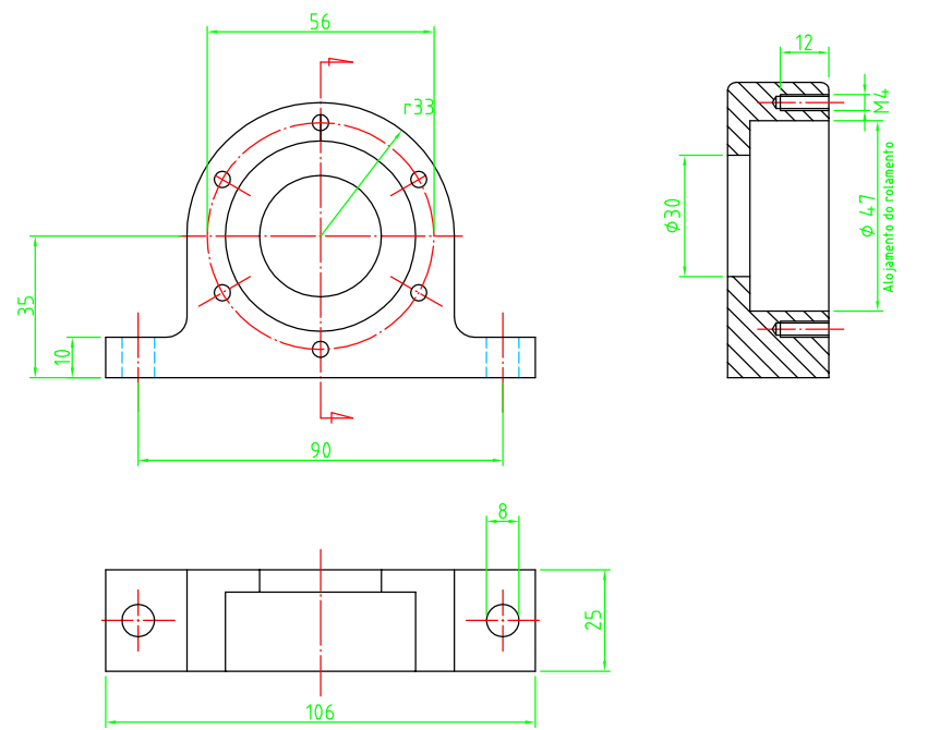
2 - Capa do mancal de rolamento
