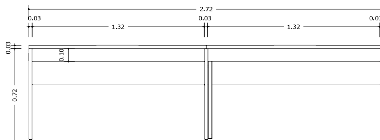
MESA COWORKING - 2 LUGARES ELEVÇÃO FRONTAL ESC 1:20
