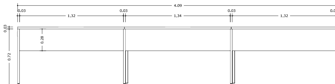
MESA COWORKING - 3 LUGARES ELEVÇÃO POSTERIOR ESC 1:20
