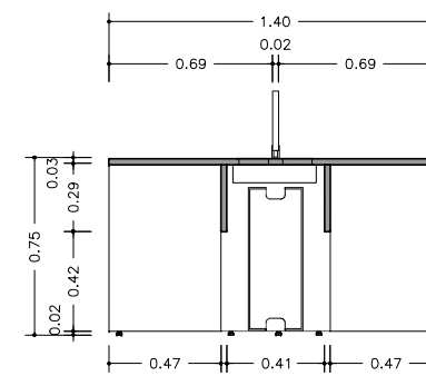
MESA COWORKING - 6 LUGARES CORTE ESC 1:25
