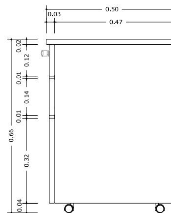
GAVETEIRO INDIVIDUAL COWORKING ELEVÇÃO LATERAL ESC 1:10
