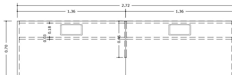
MESA COWORKING - 2 LUGARES PLANTA ESC 1:20
