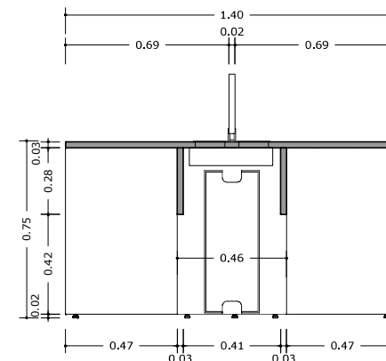
MESA COWORKING - 4 LUGARES CORTE ESC 1:20
