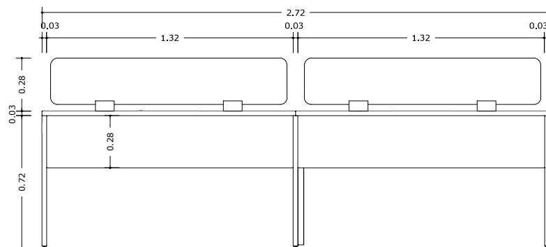
MESA COWORKING - 4 LUGARES ELEVÇÃO FRONTAL ESC 1:20
