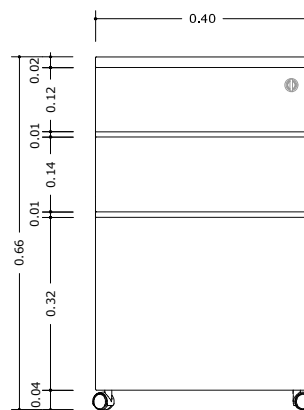
GAVETEIRO INDIVIDUAL COWORKING ELEVÇÃO FRONTAL ESC 1:10
