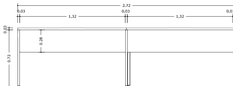
MESA COWORKING - 2 LUGARES ELEVÇÃO POSTERIOR ESC 1:20
