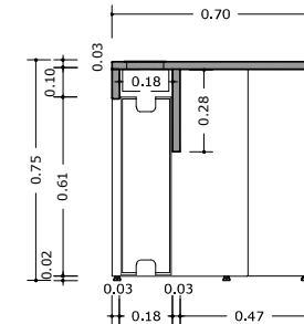
MESA COWORKING - 3 LUGARES CORTE ESC 1:20
