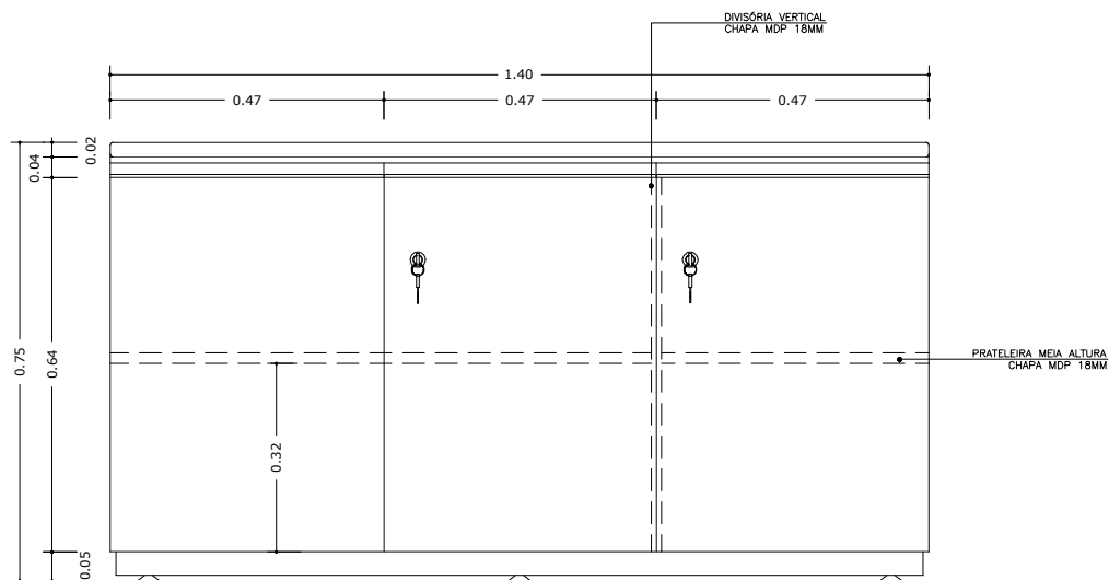
ARMÁRIO BAIXO COWORKING ELEVÇÃO FRONTAL ESC 1:10
