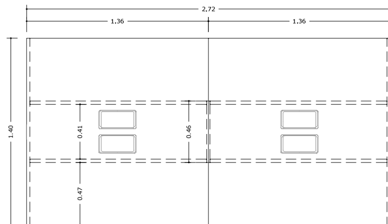
MESA COWORKING - 4 LUGARES PLANTA ESC 1:20
