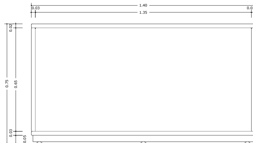
ARMÁRIO BAIXO COWORKING ELEVÇÃO POSTERIOR ESC 1:10
