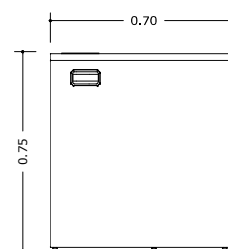
MESA COWORKING - 2 LUGARES ELEVÇÃO LATERAL ESC 1:20
