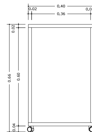
GAVETEIRO INDIVIDUAL COWORKING ELEVÇÃO POSTERIOR ESC 1:10
