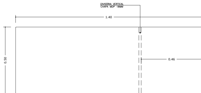
ARMÁRIO BAIXO COWORKING PLANTA ESC 1:10
