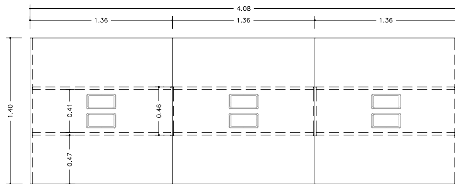
MESA COWORKING - 6 LUGARES PLANTA ESC 1:25
