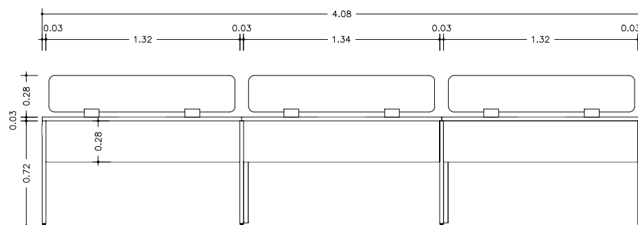
MESA COWORKING - 6 LUGARES ELEVÇÃO FRONTAL ESC 1:25
