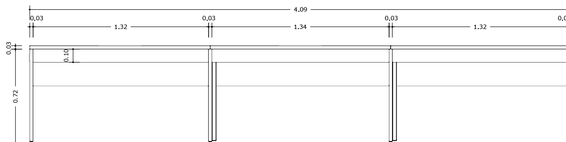
MESA COWORKING - 3 LUGARES ELEVÇÃO FRONTAL ESC 1:20
