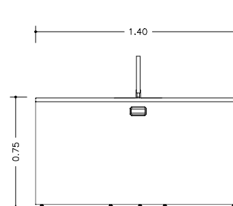
MESA COWORKING - 6 LUGARES ELEVÇÃO LATERAL ESC 1:25
