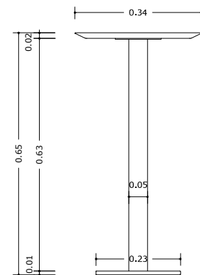
MESA DE APOIO NOTEBOOK VISTA FRONTAL ESC 1:10
