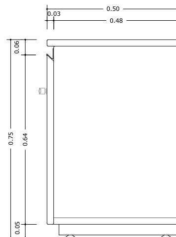
ARMÁRIO BAIXO COWORKING ELEVÇÃO LATERAL ESC 1:10
