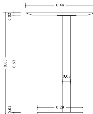
MESA DE APOIO NOTEBOOK VISTA LATERAL ESC 1:10
