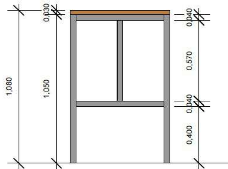
VISTA LATERAL
