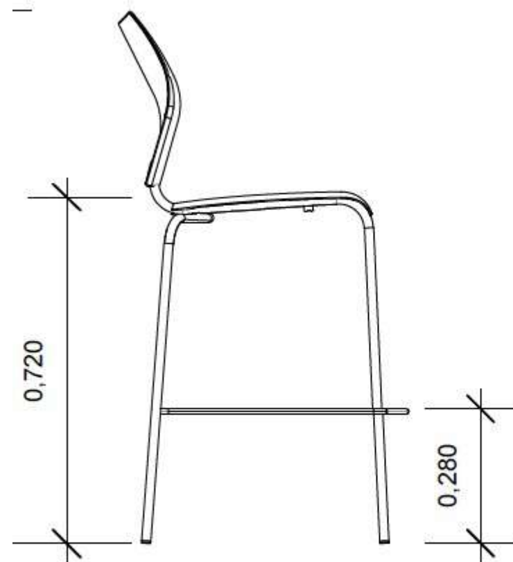
VISTA LATERAL ESC. 1/25
