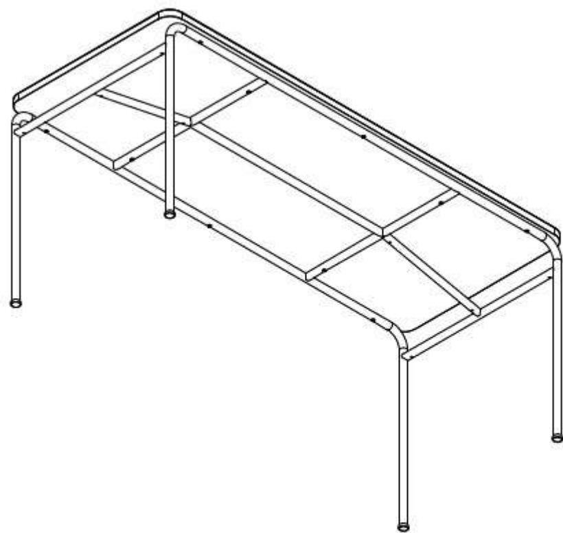
VISTA ISOMÉTRICA INFERIOR ESC. 1/25
