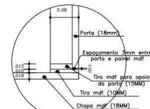
DETALHE PORTA 3 ESC 1:5
