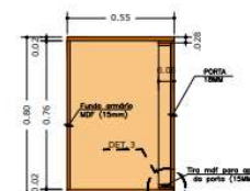
CORTE LATERAL ESC 1:20
