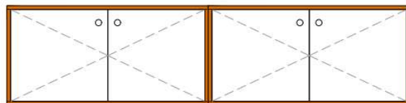
ELEVACÃO FRONTAL CONJUNTO ARMÁRIOS ESC 1:20
