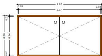
VISTA FRONTAL ESC 1:20
