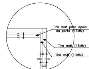
DETALHE 1 ESC 1:5
