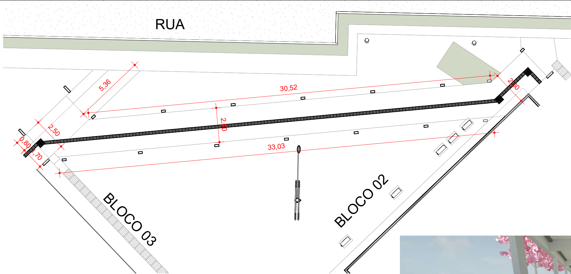
3 DETALHE - PISO BLOCO 02 AO 03 1 : 150
