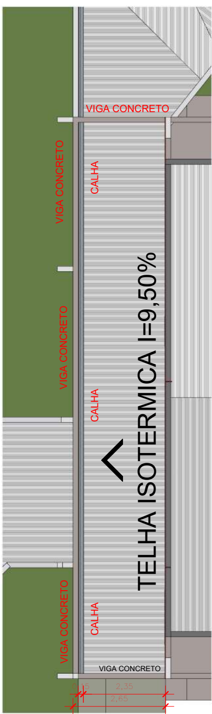
6 COBERTURA BLOCO 03 1 : 100
