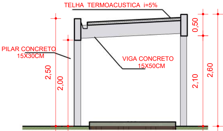
13 Corte Passarela 3-4 1 : 50
