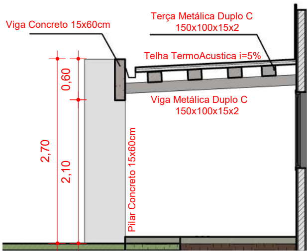
7 Corte Bloco 03 1 : 50
