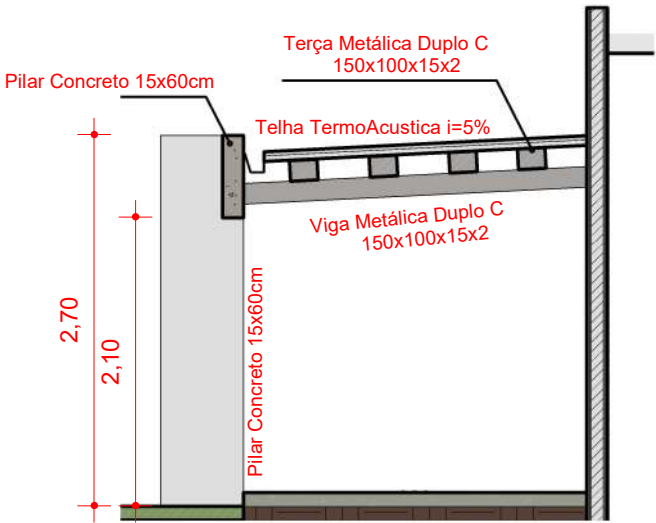
1 Corte Bloco 04 1 : 50
