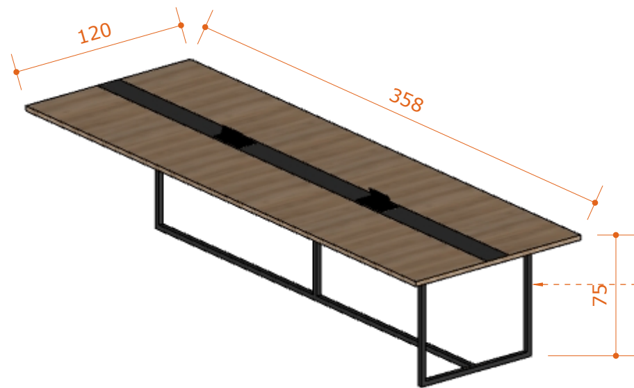
01 - MESA - PERSPEC. ESC.: 1:30
