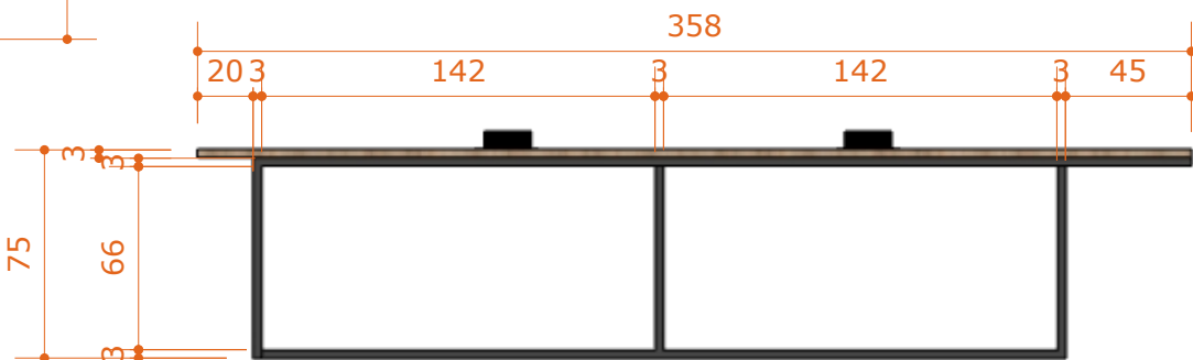
03 - MESA - LATERAL ESC.: 1:30
