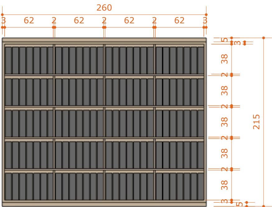
02 - ARMÁRIO - FRONTAL ESC.: 1:30
