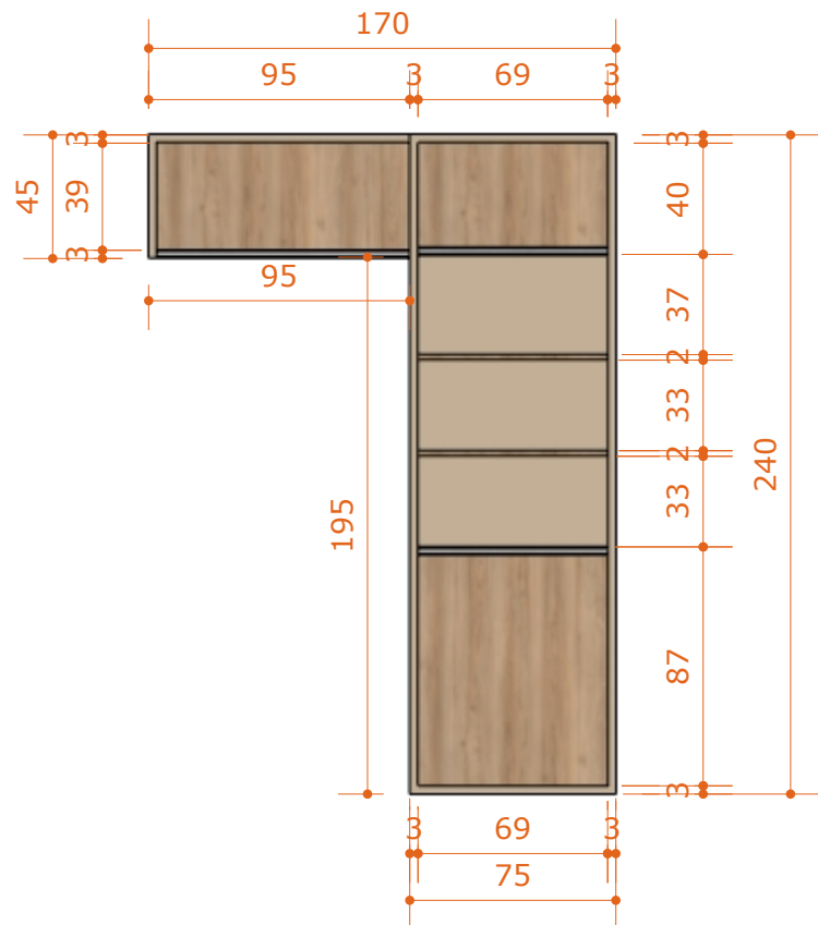
02 - VISTA FRONTAL ESC.: 1:30
