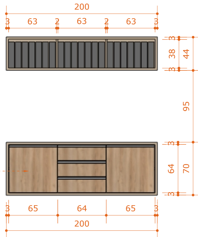
05 - ARMÁRIOS - FRONTAL ESC.: 1:30
