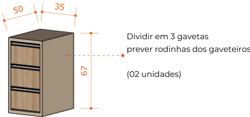
03 - GAVETEIRA - PERSPECTIVA ESC.: 1:30
