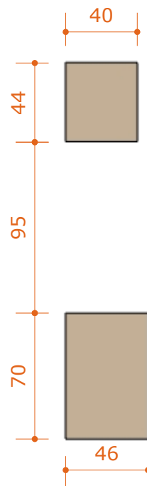
04 - ARMÁRIOS - LATERAL ESC.: 1:30
