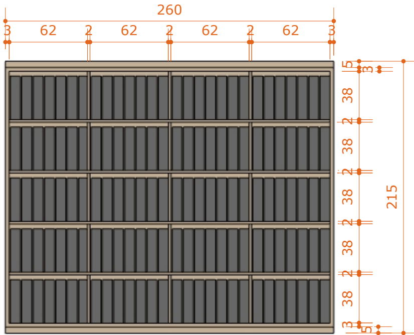
02 - ARMÁRIO - FRONTAL ESC.: 1:30
