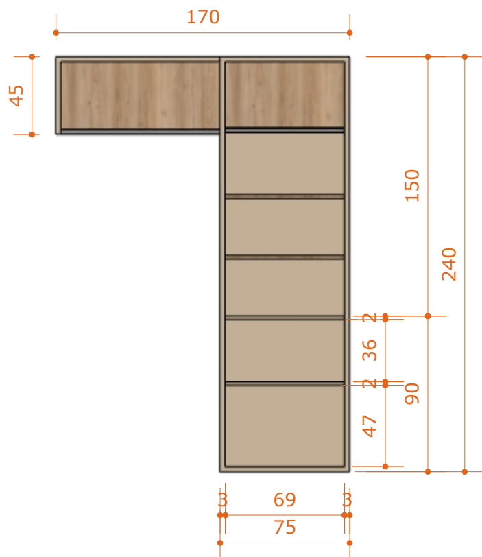
03 - VISTA LATERAL ESC.: 1:30
