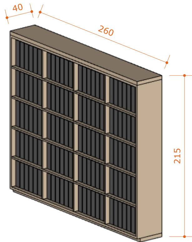
01 - ARMÁRIO - PERSPEC. ESC.: 1:30
