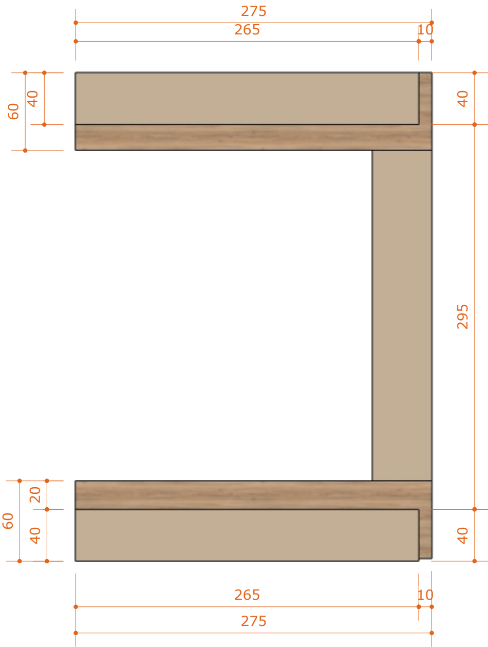
01 - ARMÁRIOS E MESA - SUPERIOR ESC.: 1:30
