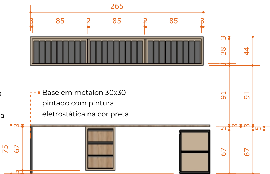
02 - ARMÁRIOS E MESA - FRONTAL ESC.: 1:30
