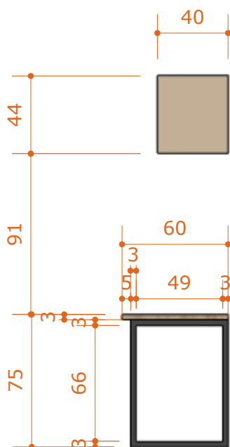
03 - ARMÁRIOS E MESA - LATERAL ESC.: 1:30
