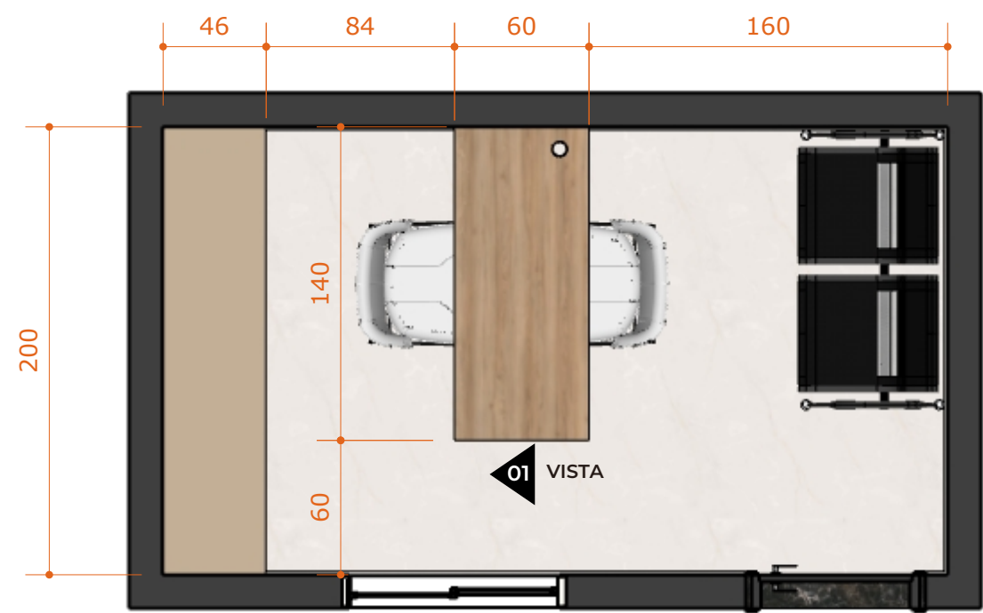
01 - PLANTA BAIXA ESC.: 1:30
