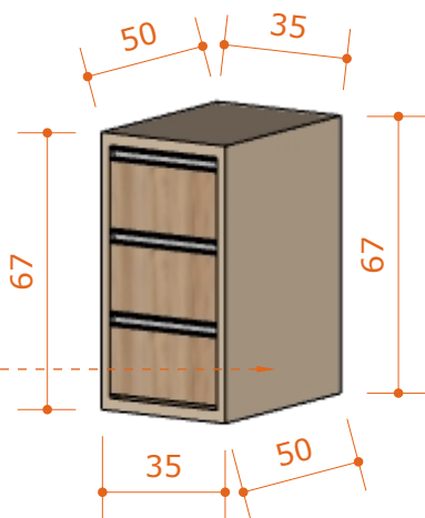
05 - GAVETEIRO - PERSPECTIVA ESC.: 1:30
