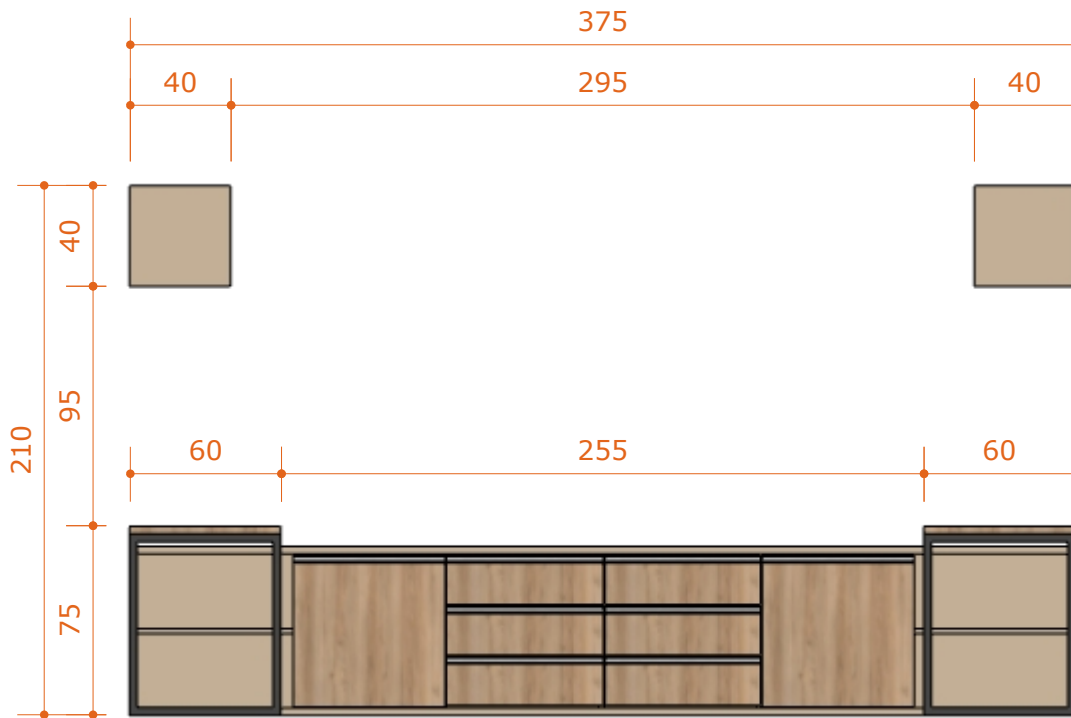
04 - ARMÁRIOS - FRONTAL ESC.: 1:30
