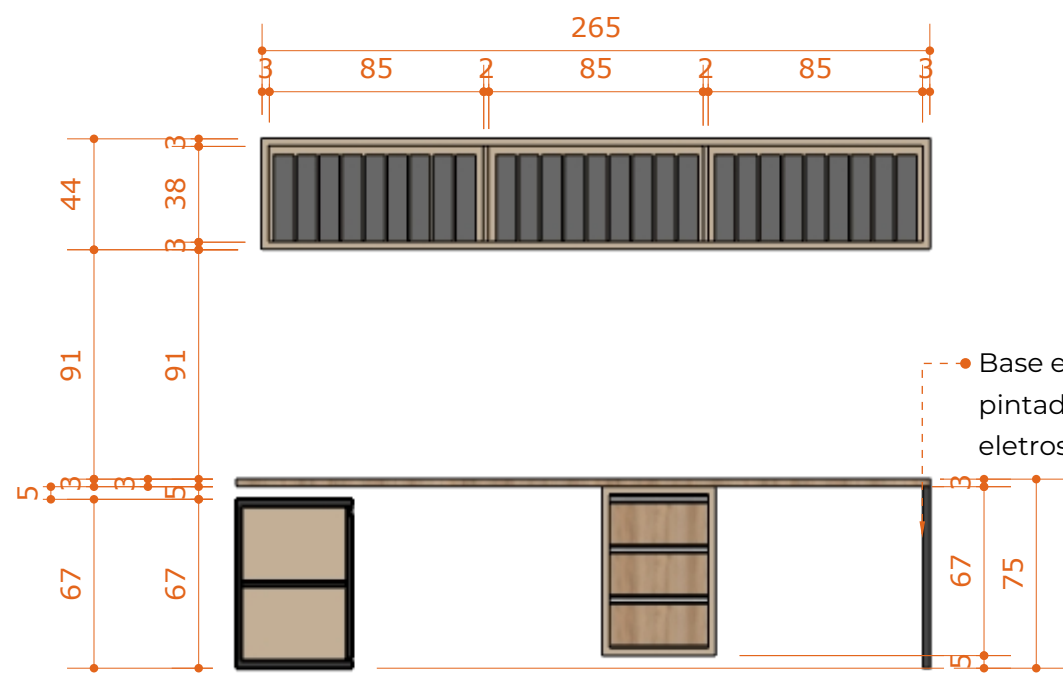
01 - ARMÁRIOS E MESA - FRONTAL ESC.: 1:30
