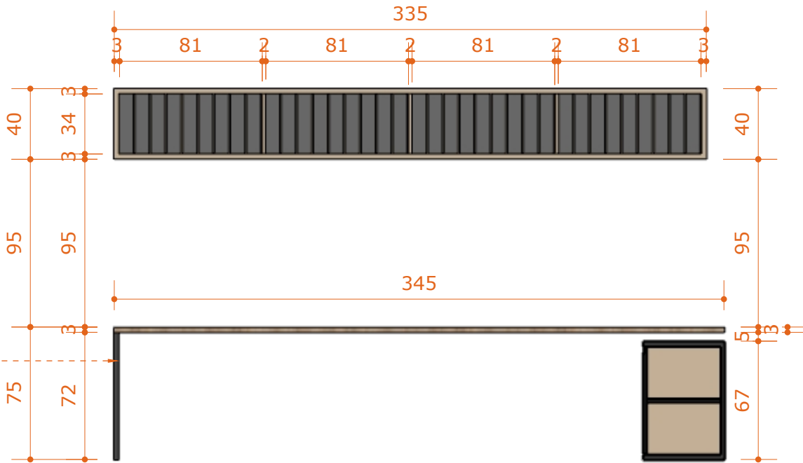
03 - ARMÁRIOS E MESA - LATERAL ESC.: 1:30
