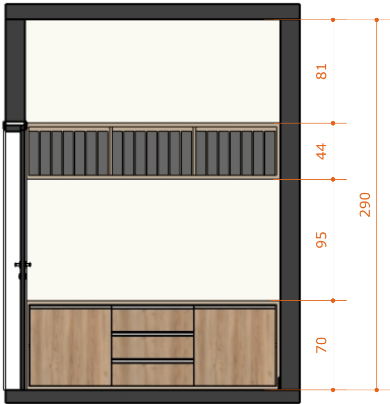
02 - VISTA 01 ESC.: 1:30
