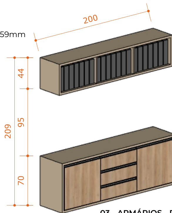
03 - ARMÁRIOS - PERSPEC. ESC.: 1:30
