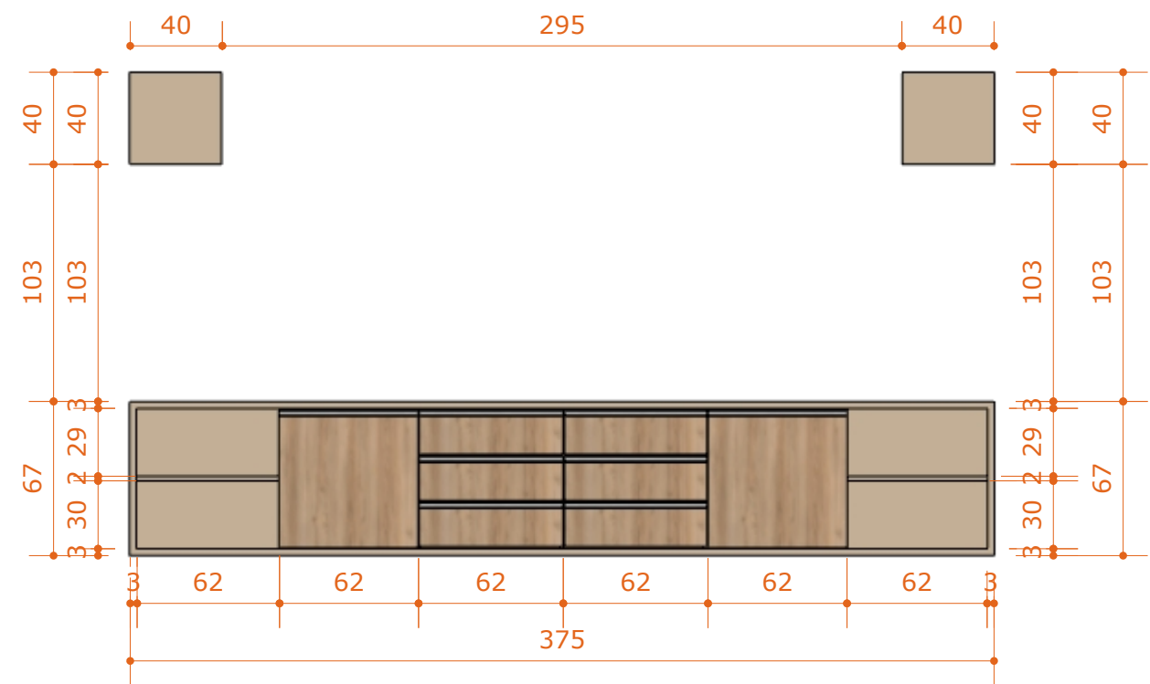
01 - ARMÁRIO - FRONTAL ESC.: 1:30
