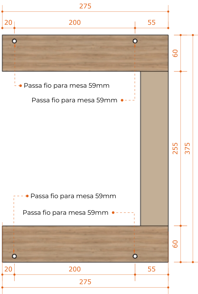
02 - ARMÁRIOS E MESA - SUPERIOR ESC.: 1:30
