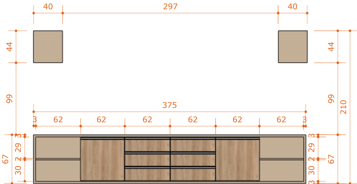
04 - ARMÁRIOS - FRONTAL ESC.: 1:30
