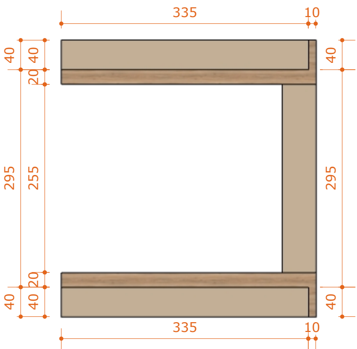
02 - ARMÁRIOS E MESA - SUPERIOR ESC.: 1:30
