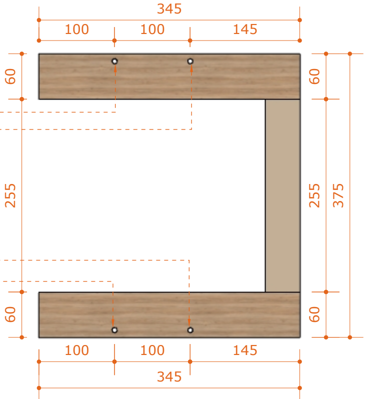
03 - ARMÁRIO E MESA - SUPERIOR ESC.: 1:30
