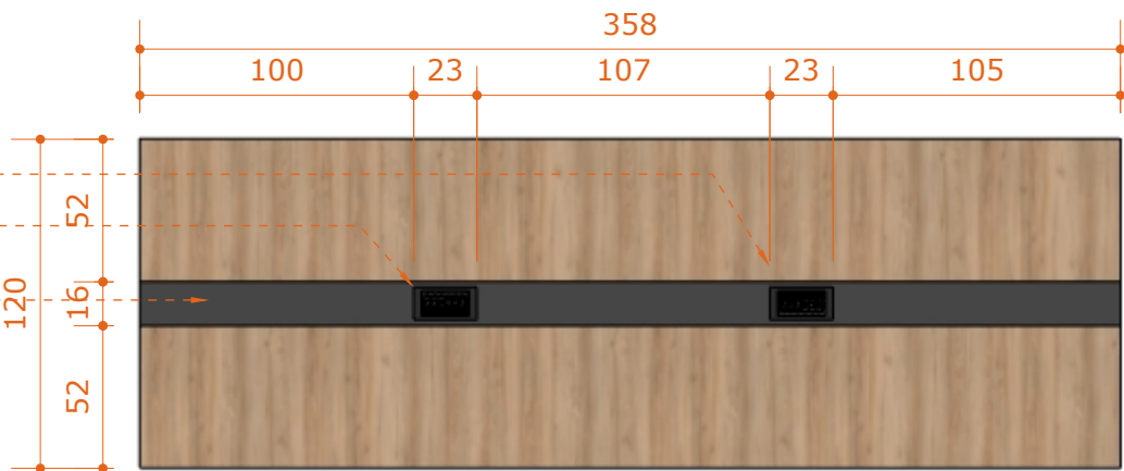
02 - MESA - SUPERIOR ESC.: 1:30
