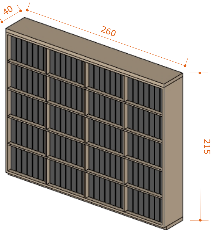
01 - ARMÁRIO - PERSPEC. ESC.: 1:30
