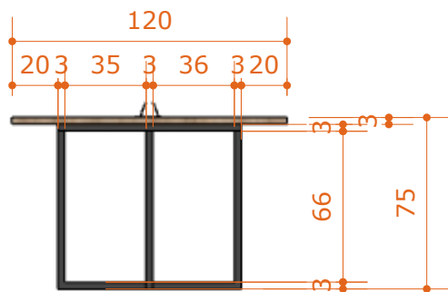
04 - MESA - FRONTAL ESC.: 1:30
