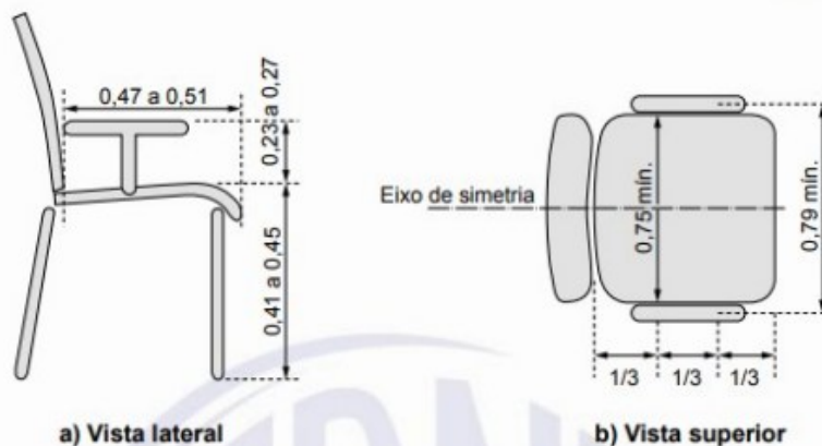
Figura 27 – Dimensões para assentos para pessoas obesas
