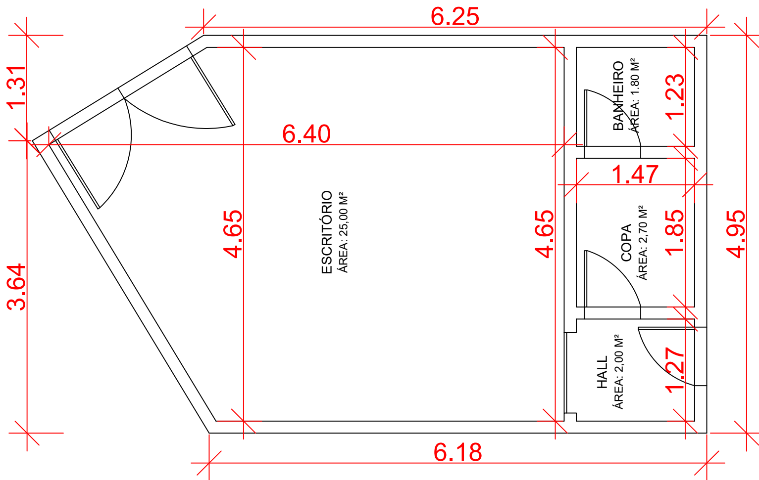
PLANTA BAIXA - SALA COMERCIAL SEM ESCALA
