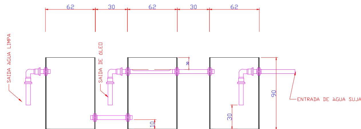
SEPARADOR DE ÓLEO CORTE - ESC. 1:25
