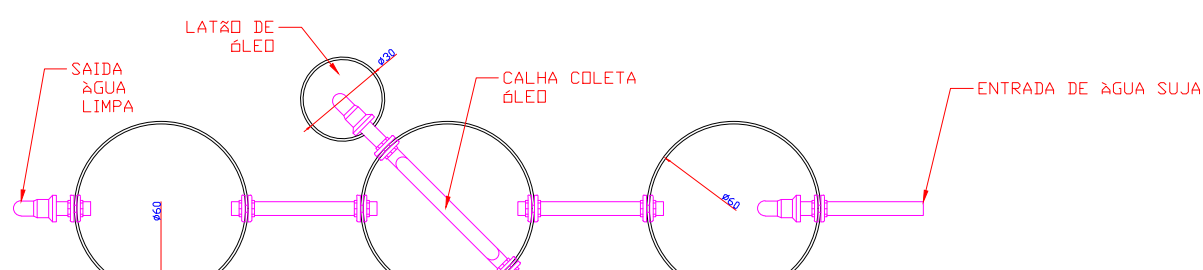
SEPARADOR DE ÓLEO Planta baixa - ESC. 1:25
