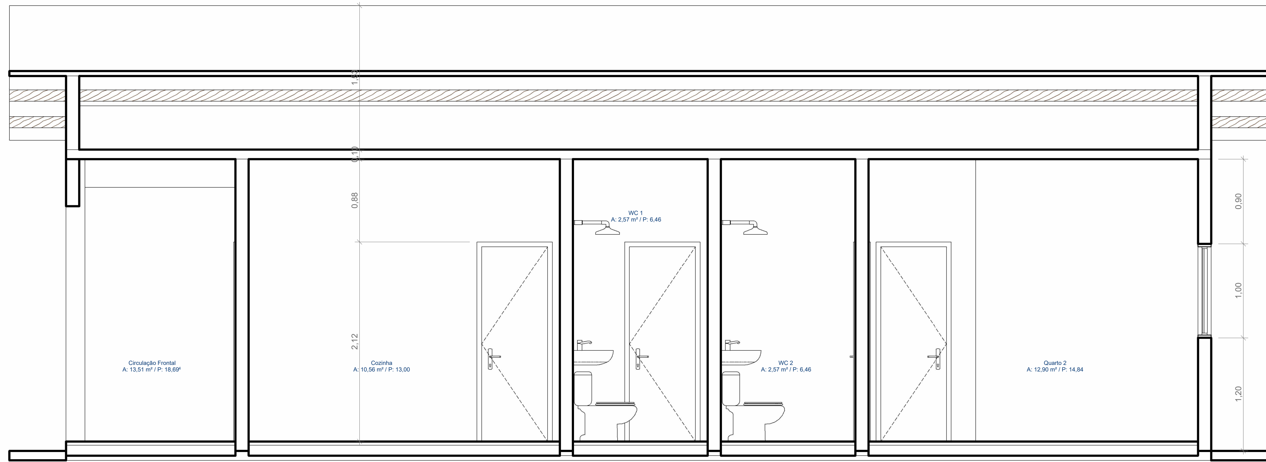
3 - Section 0 ESCALA 1 : 25
