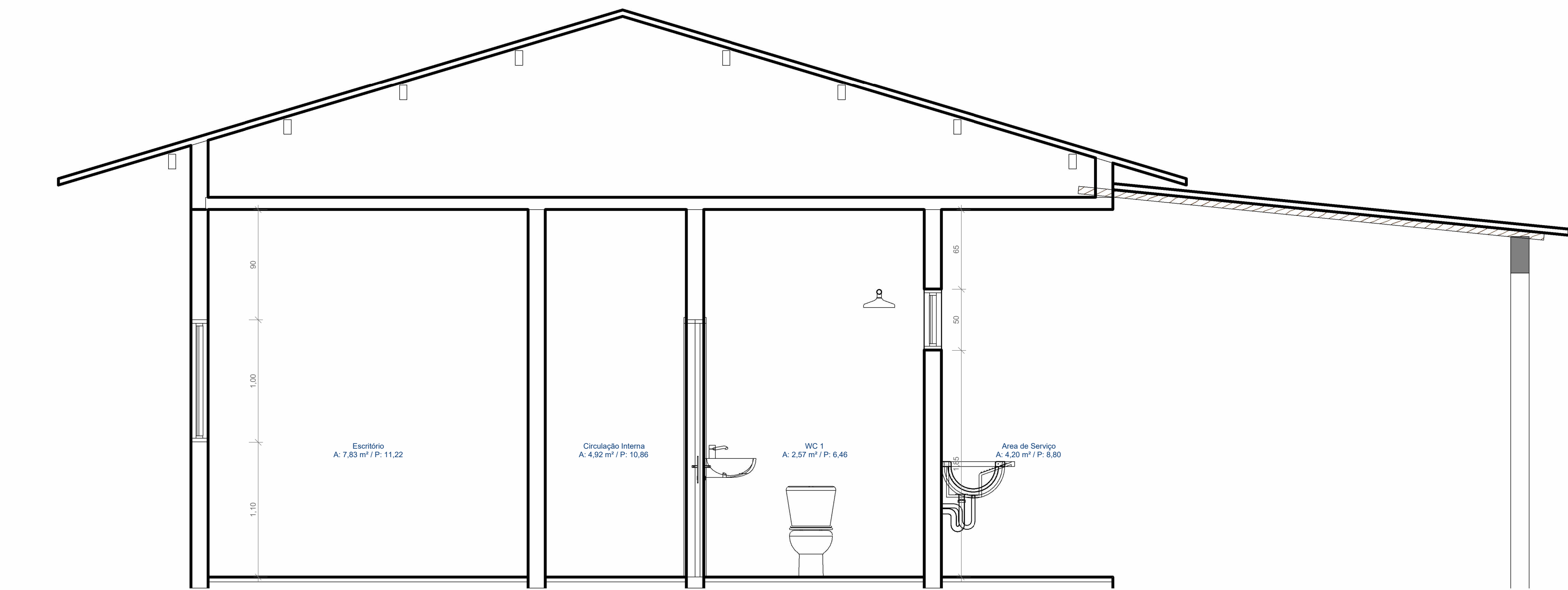
4 - Section 1 ESCALA 1 : 25
