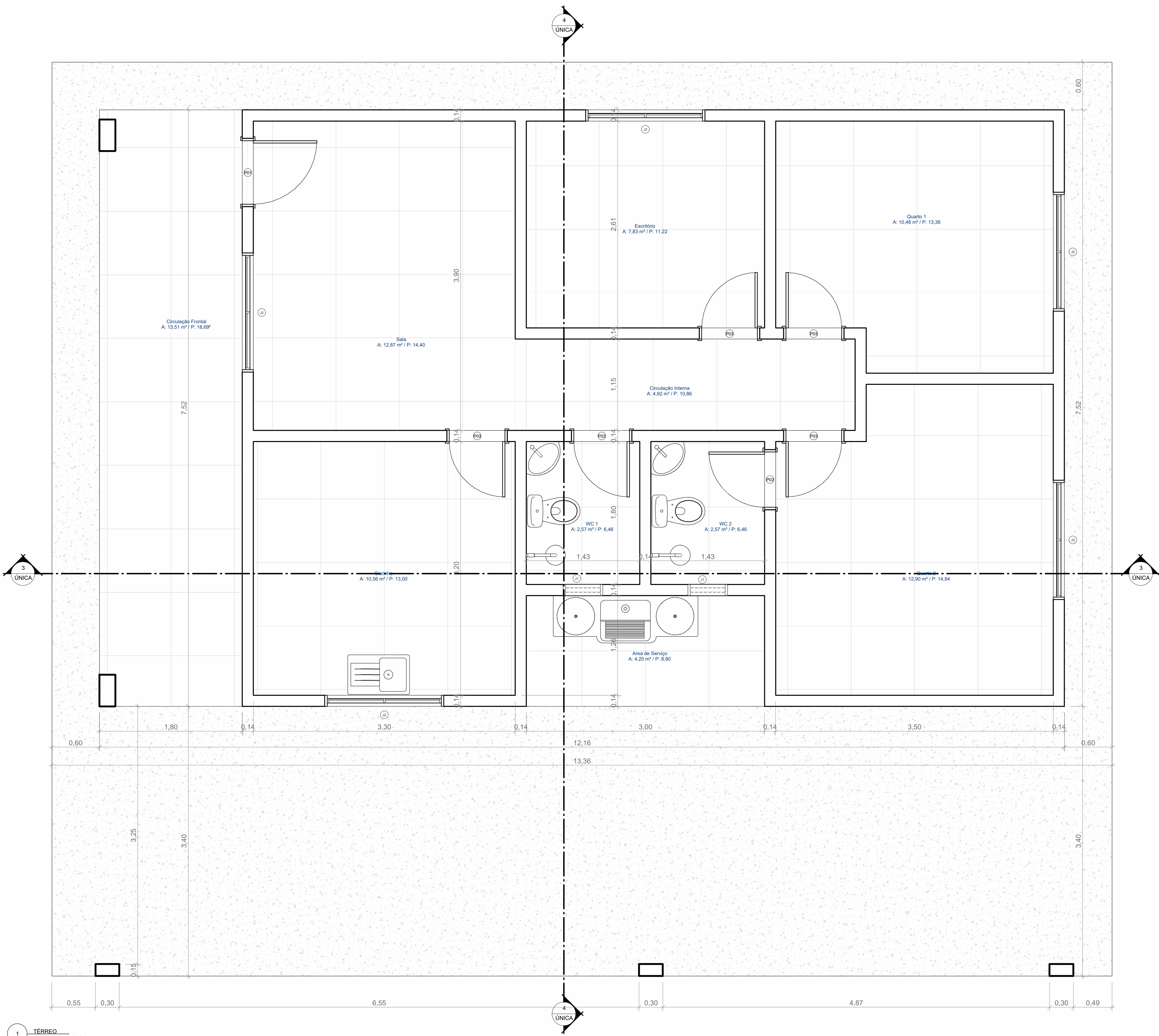
1 - TÉRREO ESCALA 1 : 25
