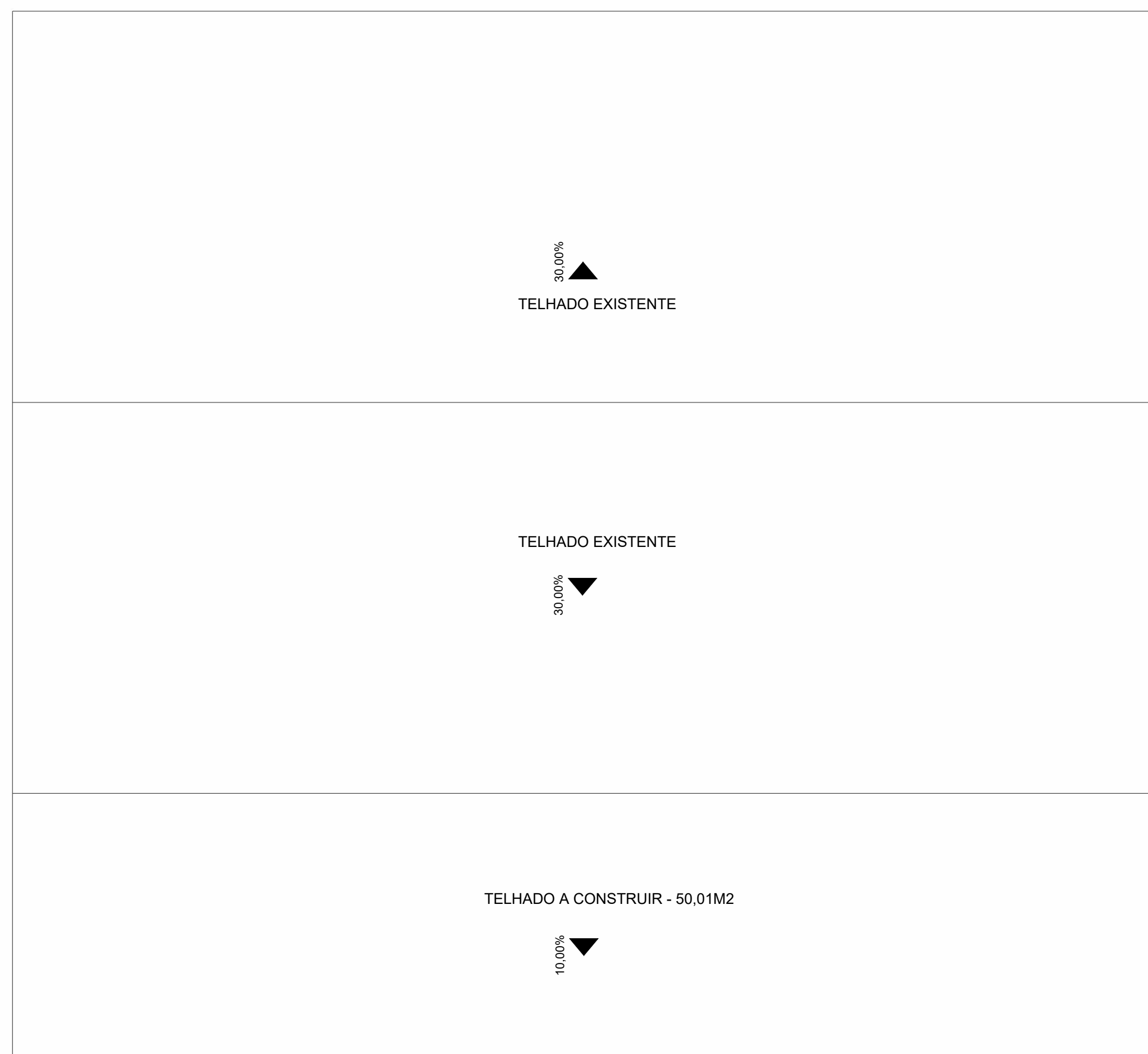
5 - COBERTURA ESCALA 1 : 50
