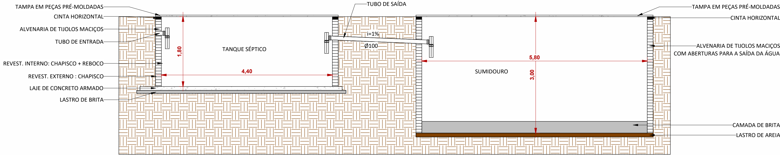
DET. FOSSA E SUMIDOURO
