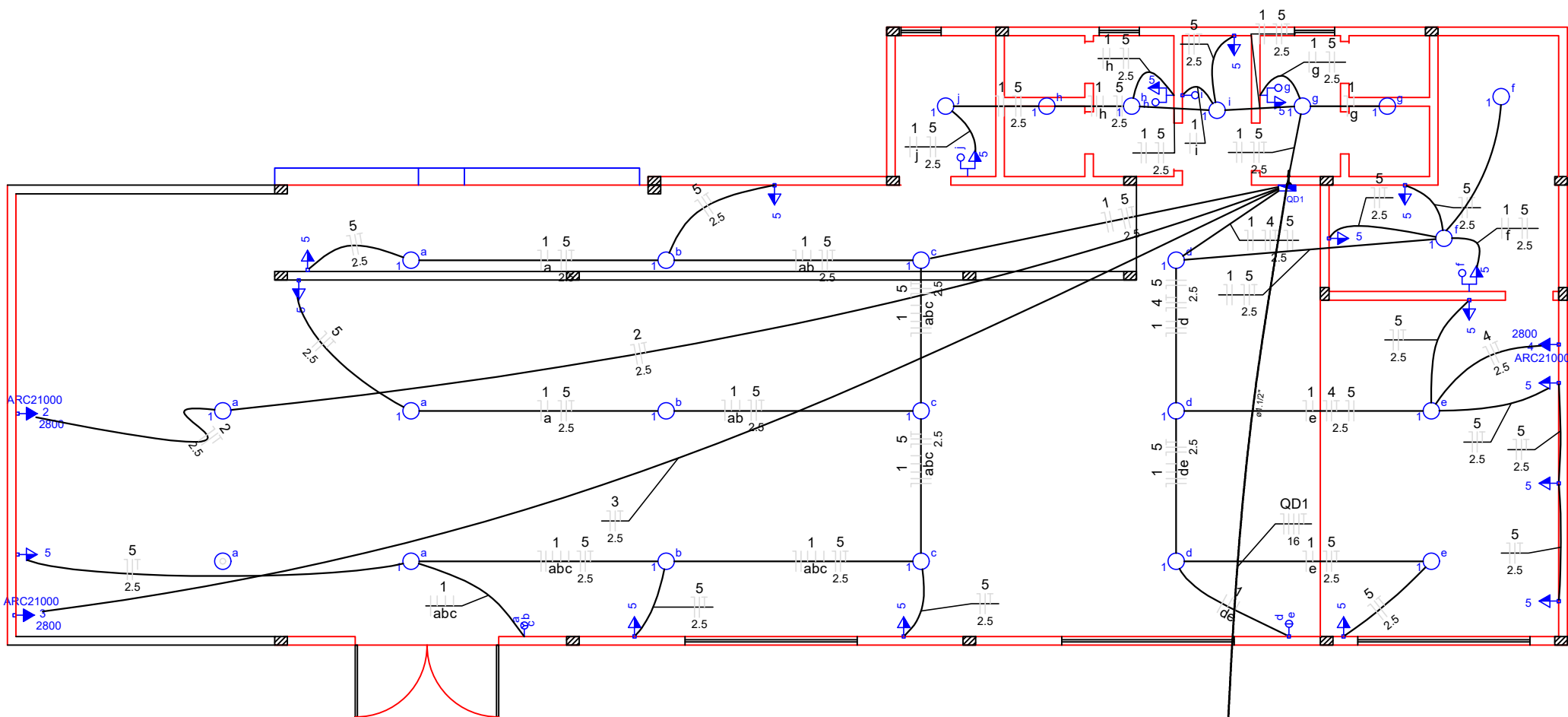
Elétrico - Pav. Superior Escala: 1/100
