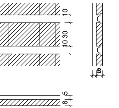
Detalhe 2 (esc. 1:30)
