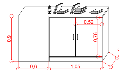
CORTE C-C
