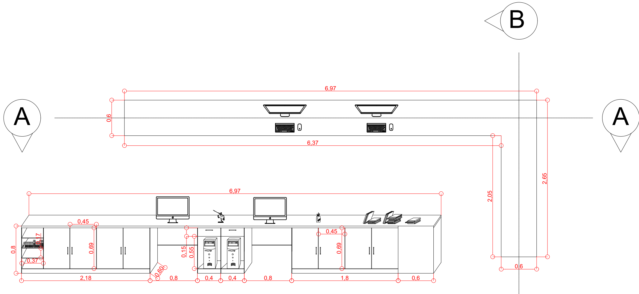
CORTE A-A
