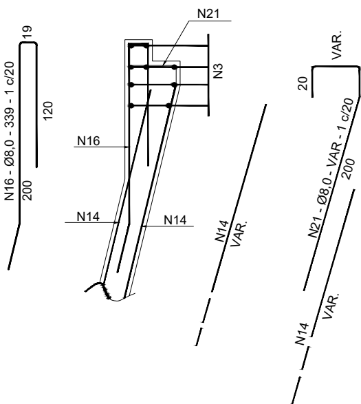
SEÇÃO 2-2 (4X) ESC. 1:50
