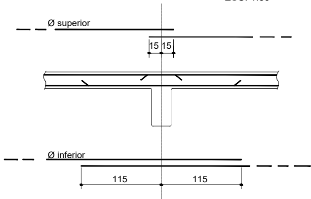
LIGAÇÃO DE BUEIROS COM AS CABECEIRAS ( LAJE INFERIOR ) ESC. 1:50
