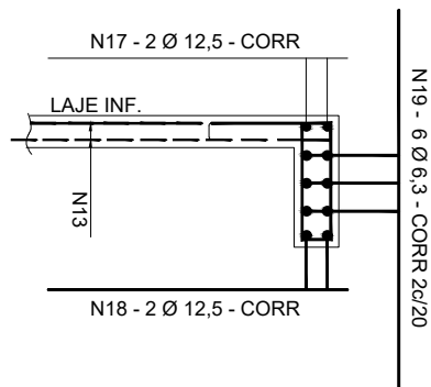
SEÇÃO DA VIGA DE TOPO DE LAJE INFERIOR ( 2X ) ESC. 1:50
