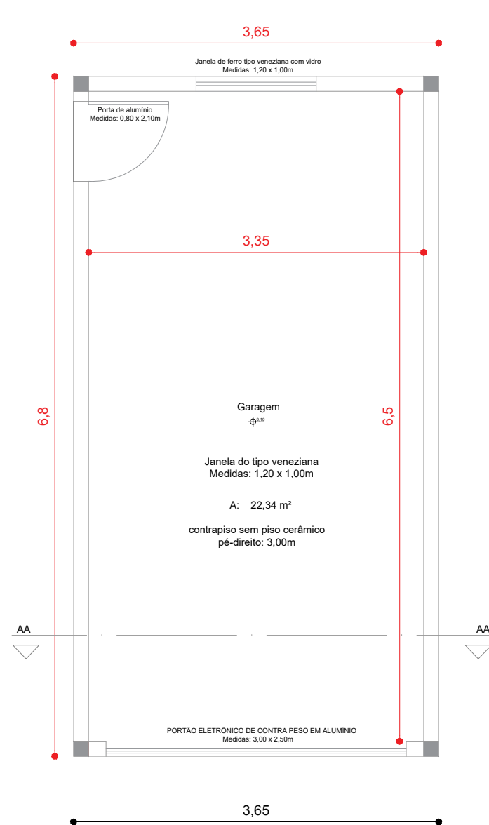
PLANTA BAIXA
