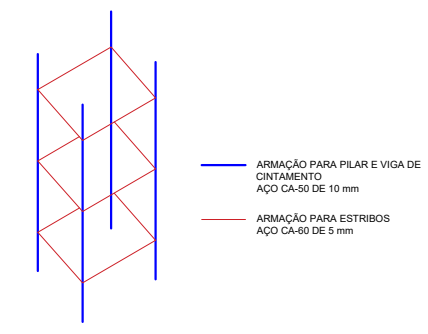
DETALHE FERROS E ESTRIBO
