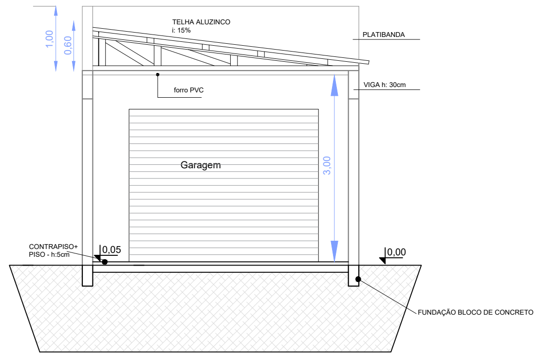
CORTE AA'
