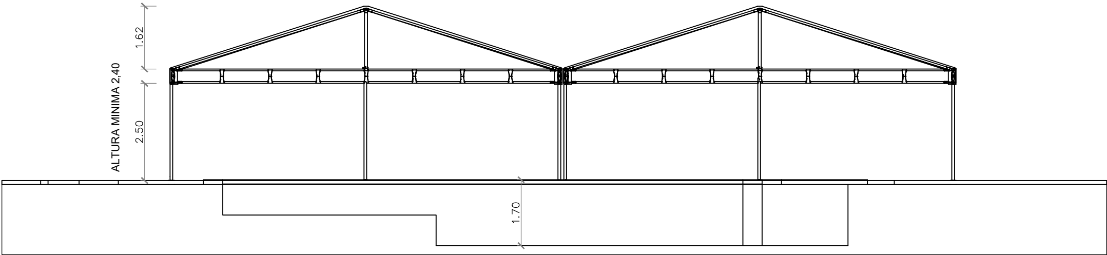
1.0 CORTE B-B Escala 1/100
