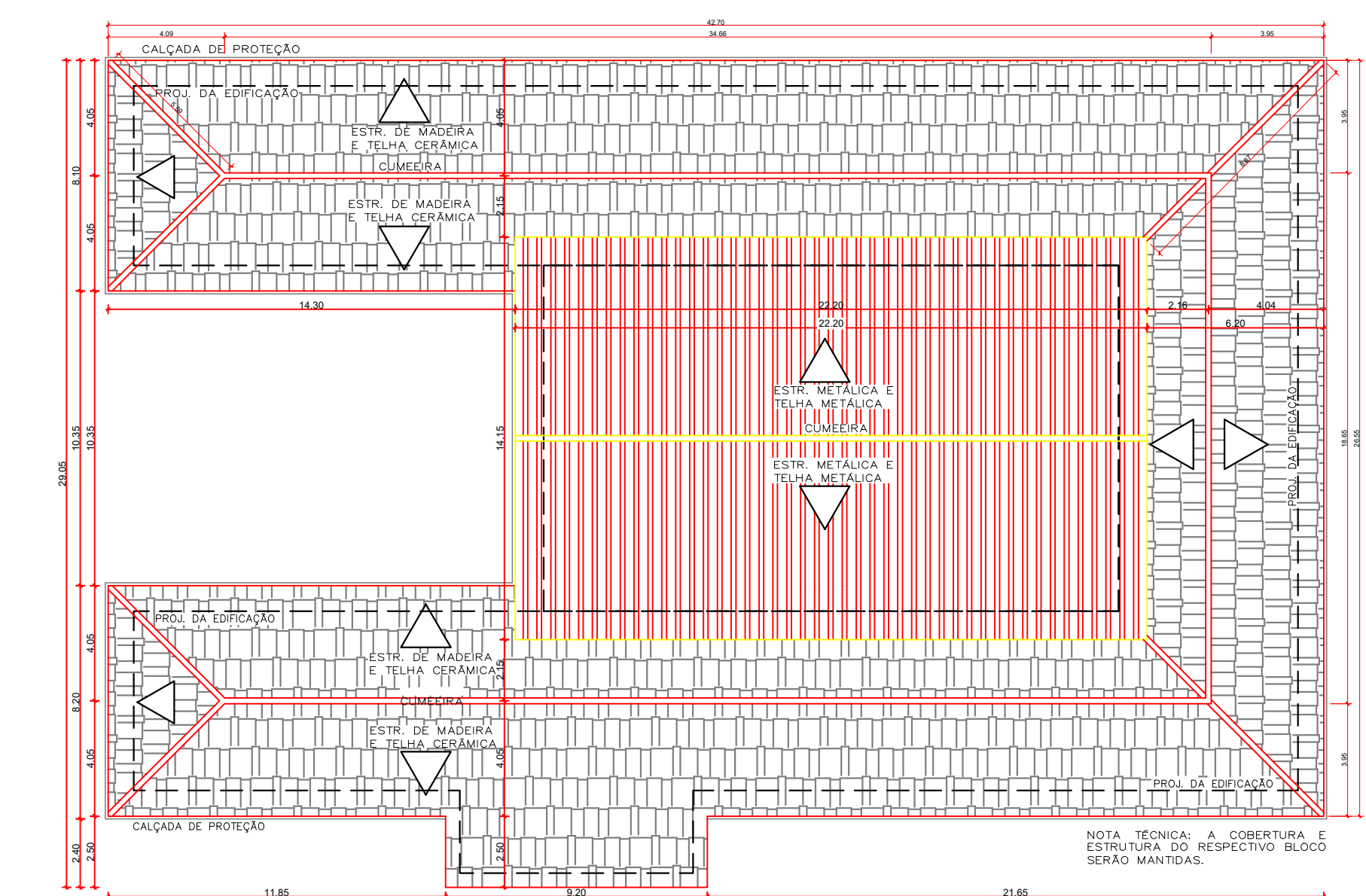
COBERTURA - LEVANTADA ESCALA: 1:200
