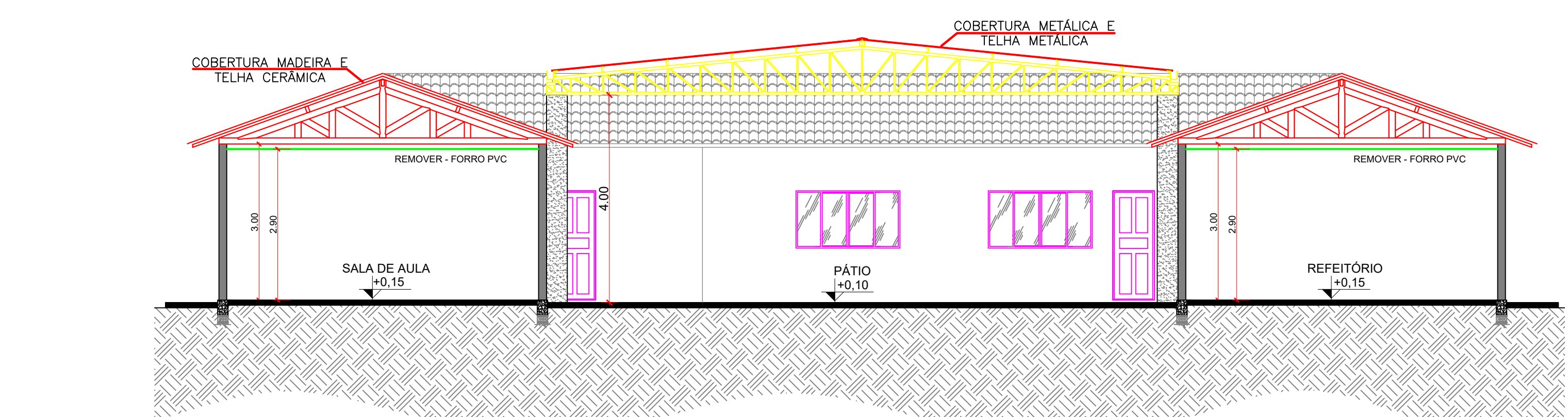
CORTE B'B ESCALA: 1:75
