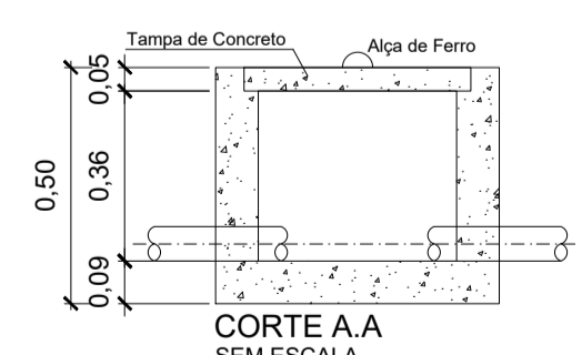
CORTE A-A SEM ESCALA
