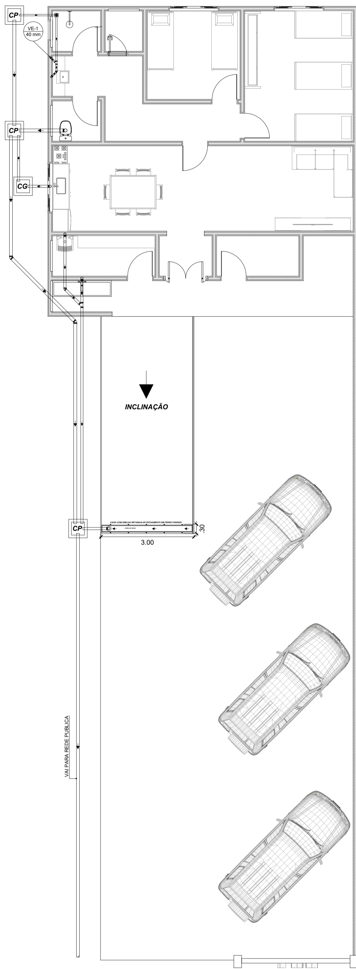
DISTRIBUIÇÃO SANITÁRIA ESCALA 1:75
