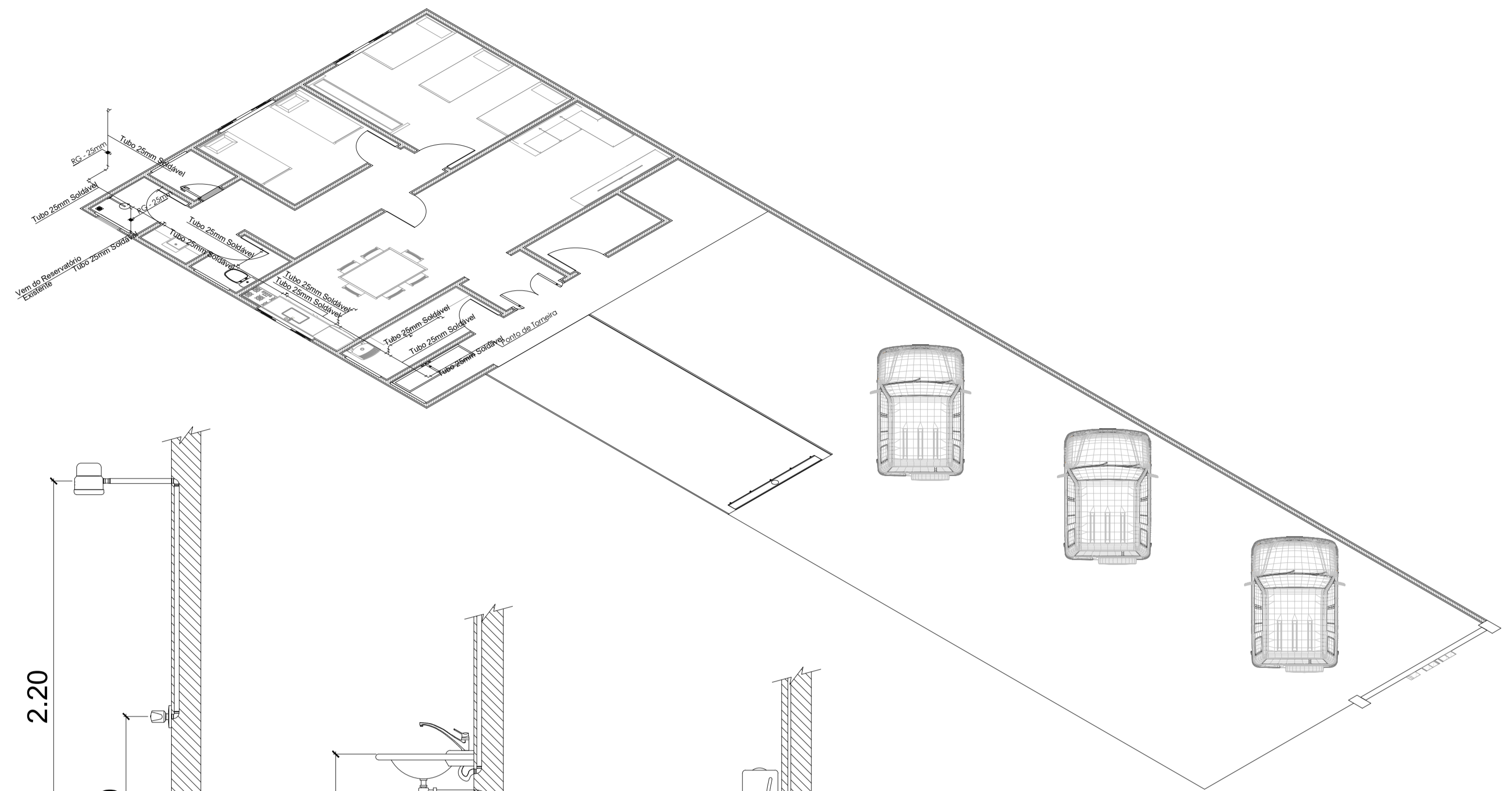
DETALHE ISOMÉTRICO - HIDRÁULICO SEM ESCALA
