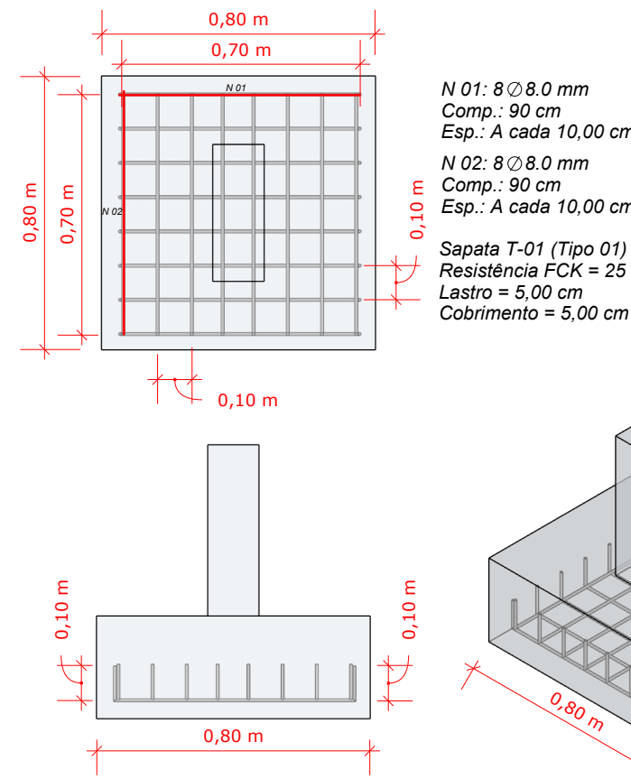
ESPECIFICAÇÕES SAPATA T-01
