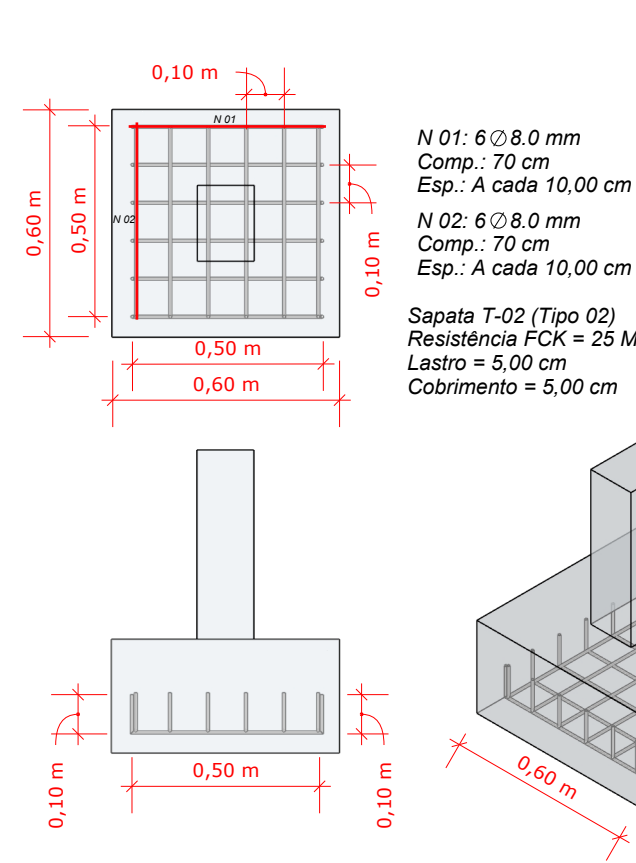
ESPECIFICAÇÕES SAPATA T-02
