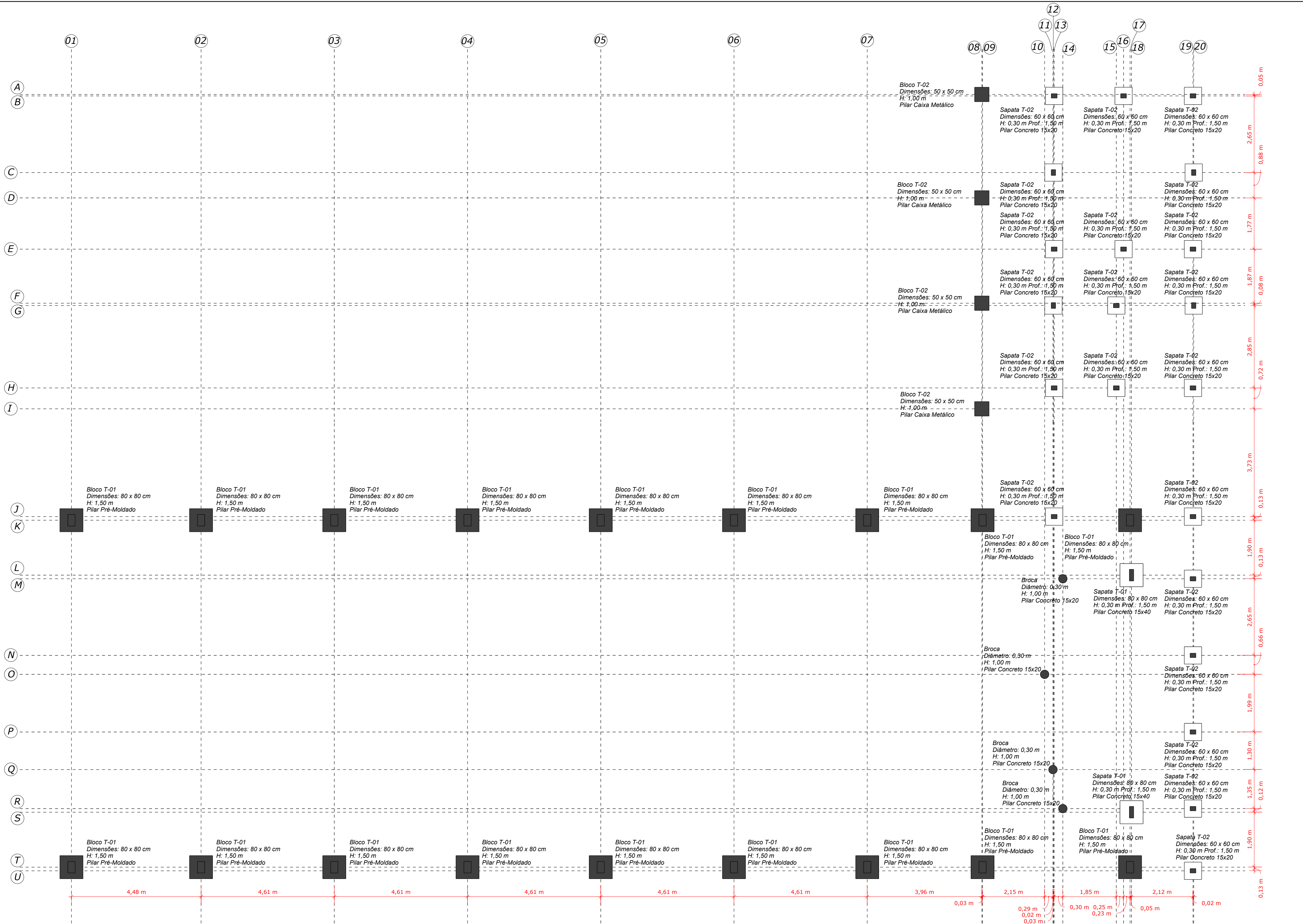
LOCAÇÃO FUNDAÇÃO - BARRACÃO
