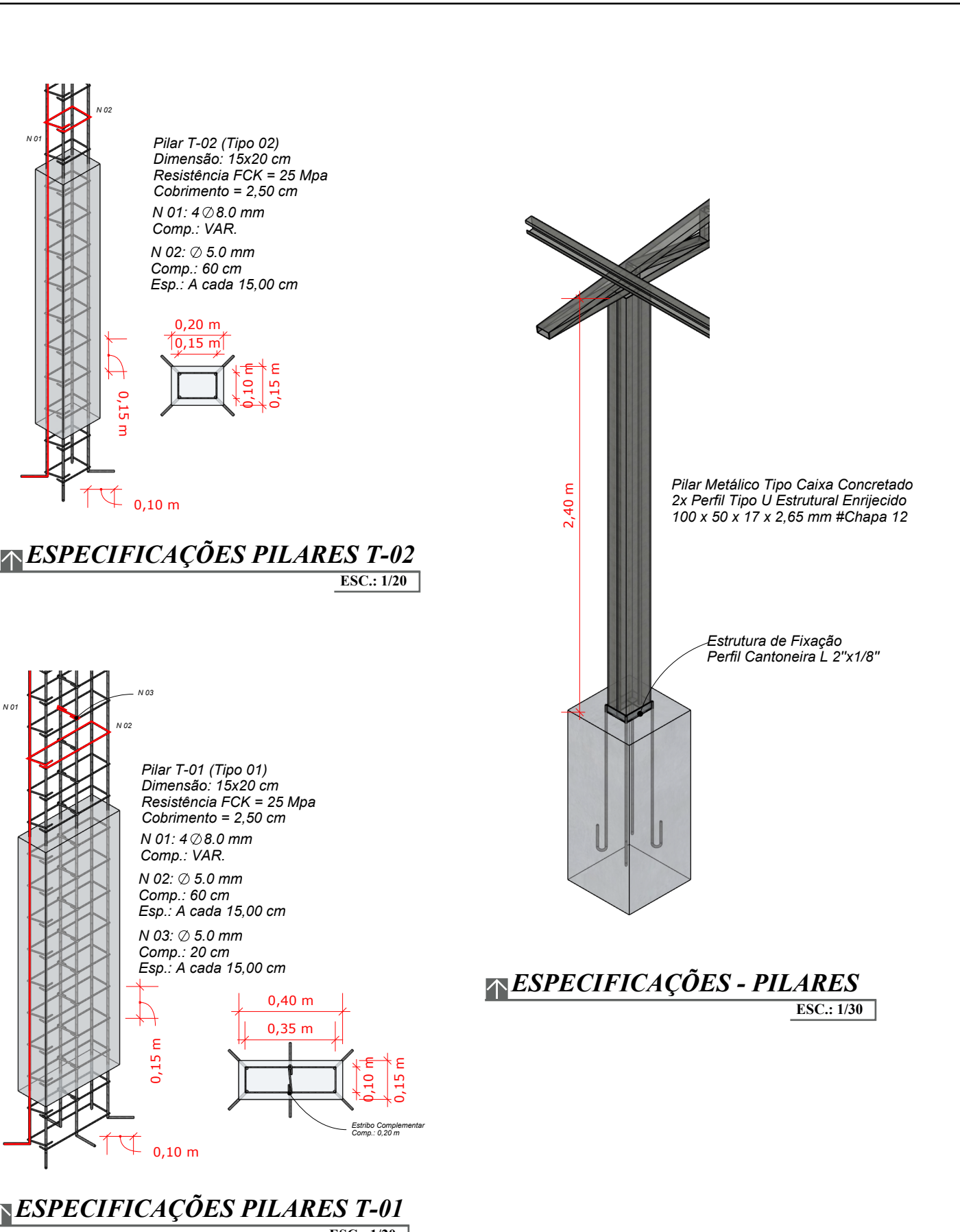
ESPECIFICAÇÕES PILARES T-01
