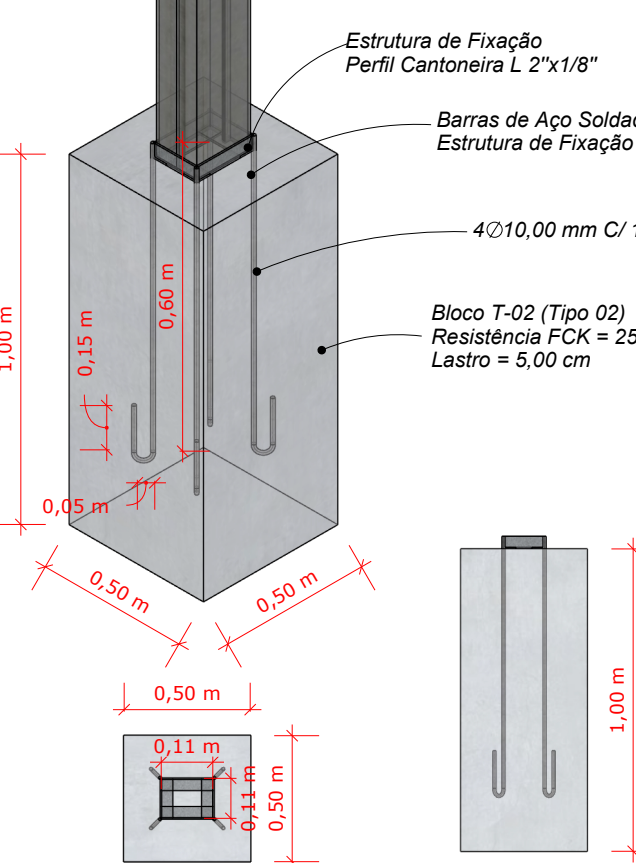
ESPECIFICAÇÕES BLOCO T-02
