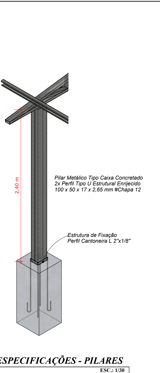
ESPECIFICAÇÕES PILARES T-02
