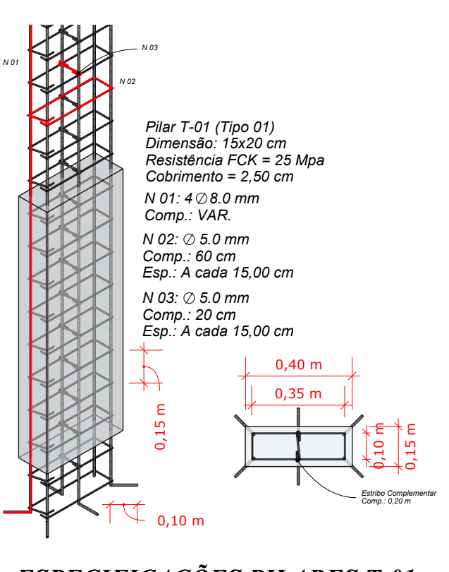
ESPECIFICAÇÕES PILARES T-01
