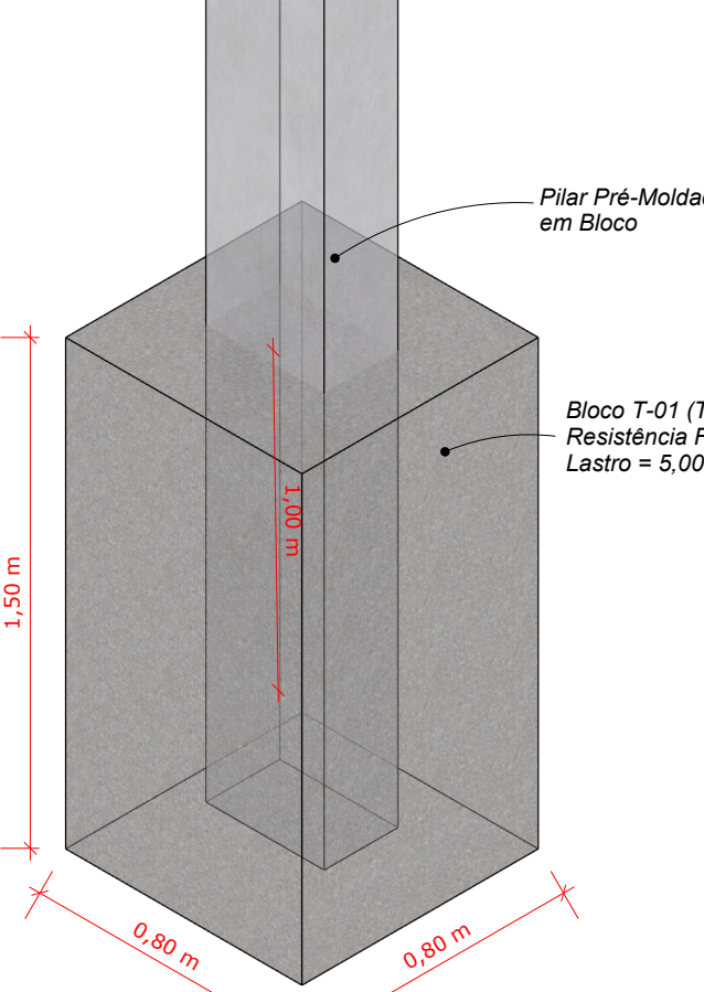
ESPECIFICAÇÕES BLOCO T-01
