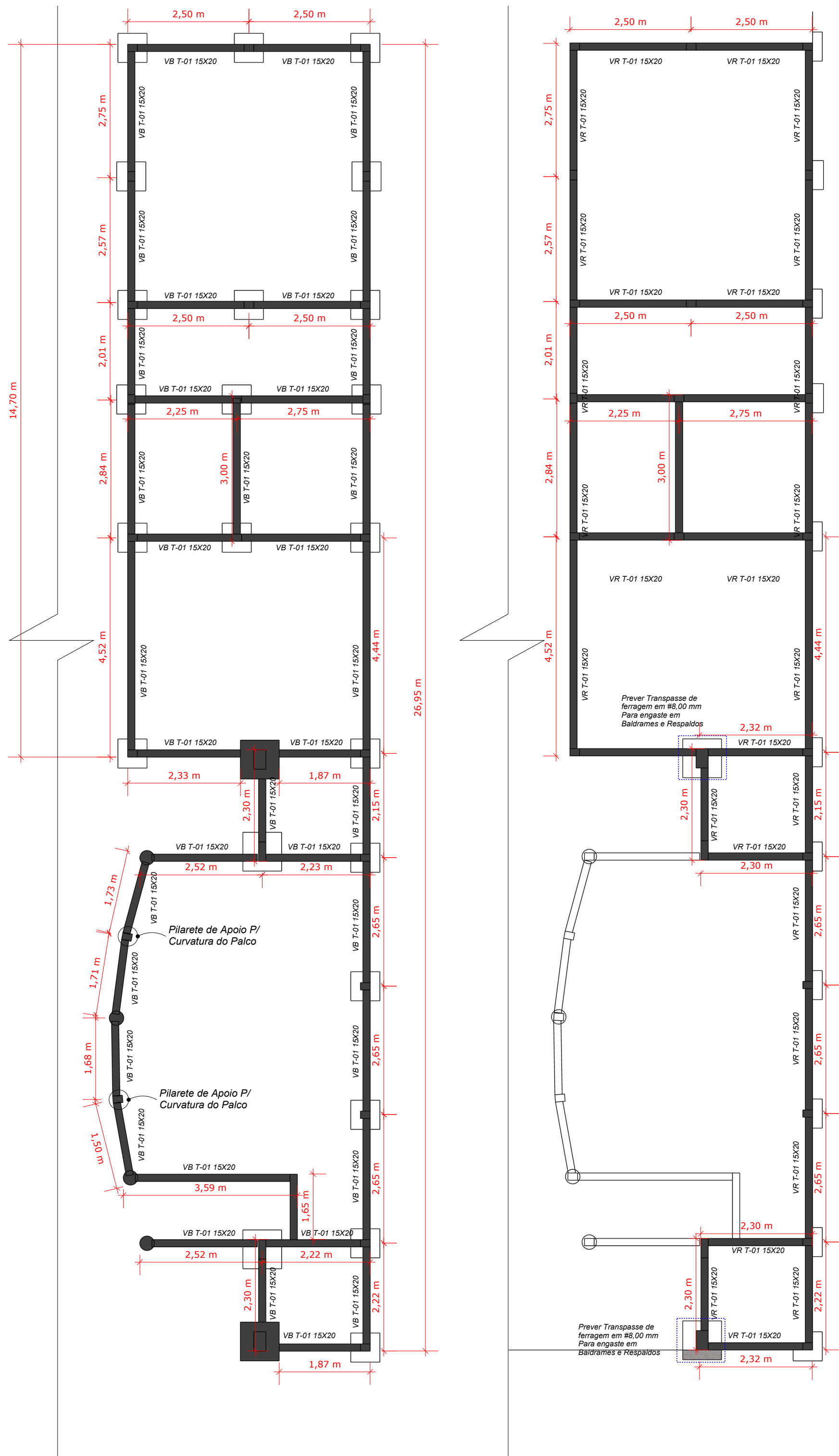
LOCAÇÃO BALDRAMES - BARRACÃO ESC.: 1/75
