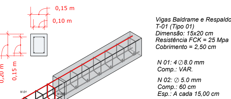
ESPECIFICAÇÕES VIGAS BALDRAME E RESPALDO T-01 ESC.: 1/20
