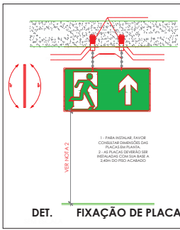
DET. FIXAÇÃO DE PLACA
