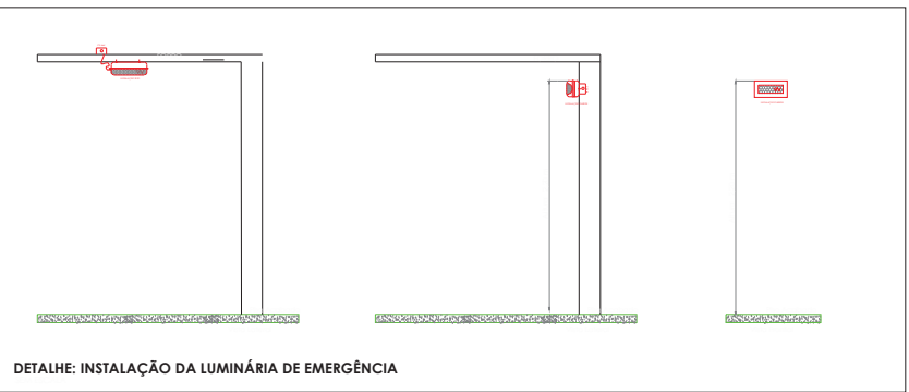
DETALHE: INSTALAÇÃO DA LUMINÁRIA DE EMERGÊNCIA
