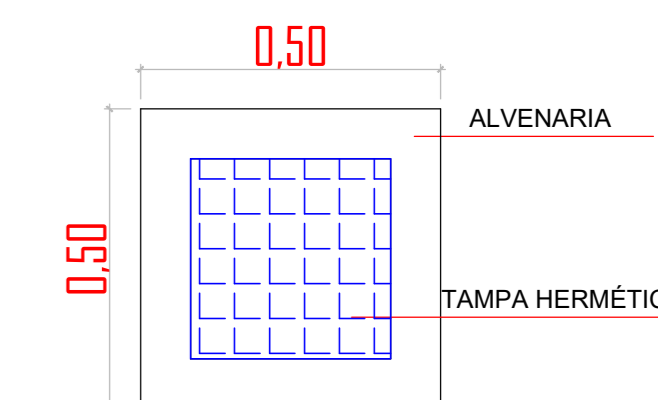
PLANTA BAIXA - CAIXA DA VÁLV. RETENÇÃO 1:100
