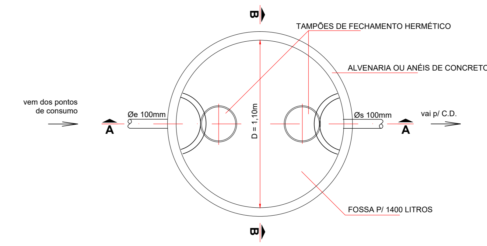
PLANTA DA FOSSA SÉPTICA 1:20
