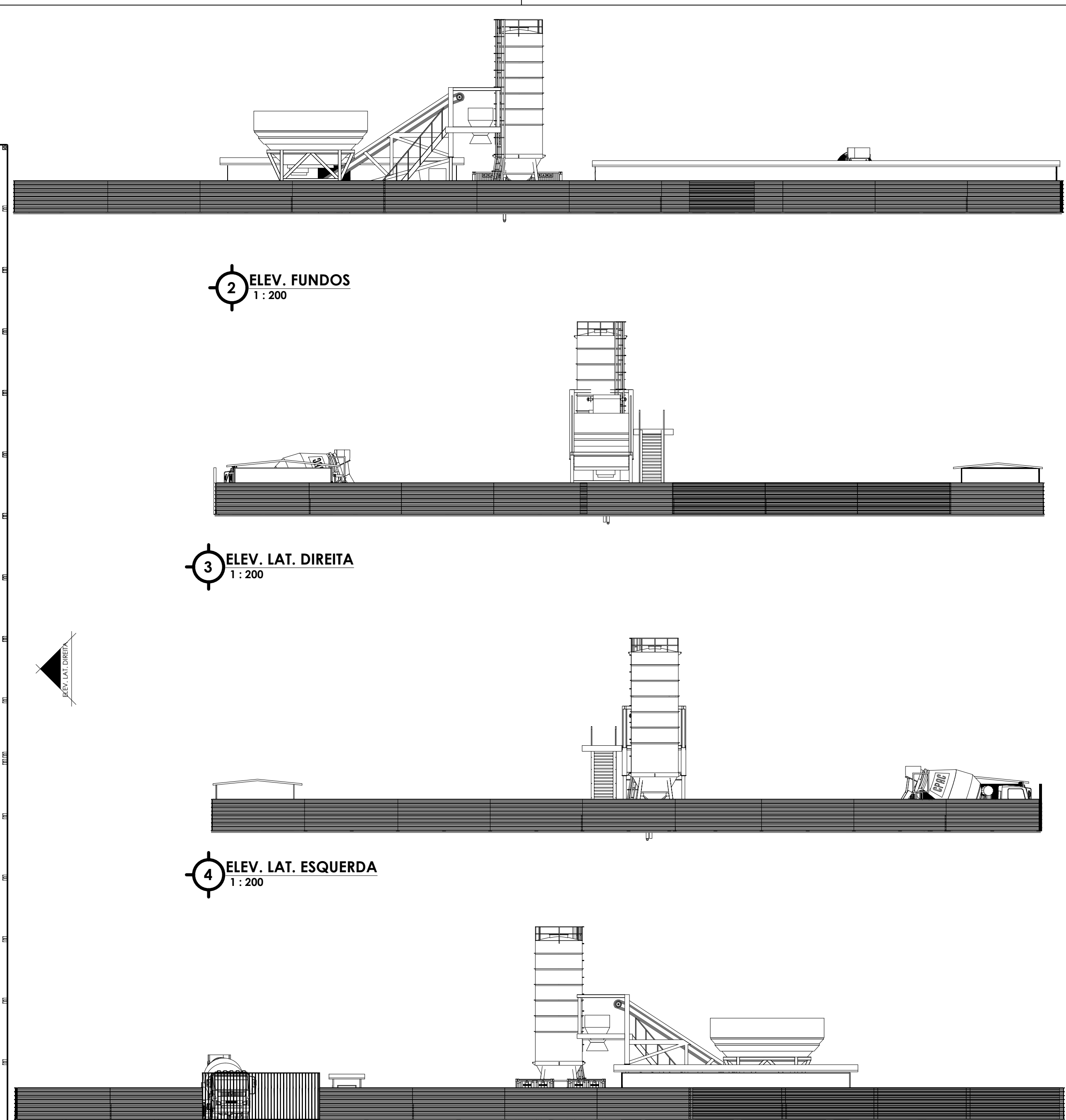
5 ELEV. FRONTAL 1 : 200
