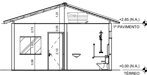
8 CORTE AA 1 : 50
