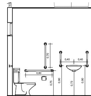
6 CORTE CC - Banho 1 : 30
