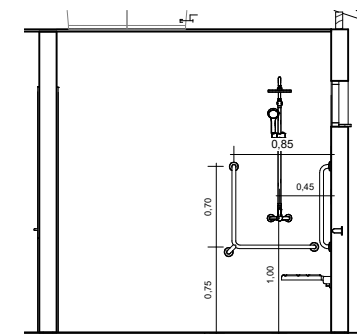
4 CORTE AA - Banho 1 : 30
