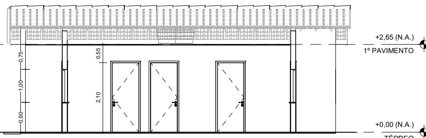
9 CORTE BB 1 : 50
