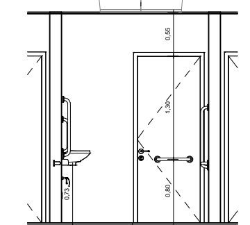
7 CORTE DD - Banho 1 : 30
