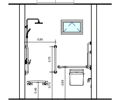
5 CORTE BB - Banho 1 : 30
