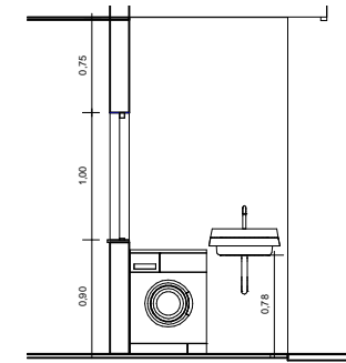
3 CORTE LAVATÓRIO 1 : 30
