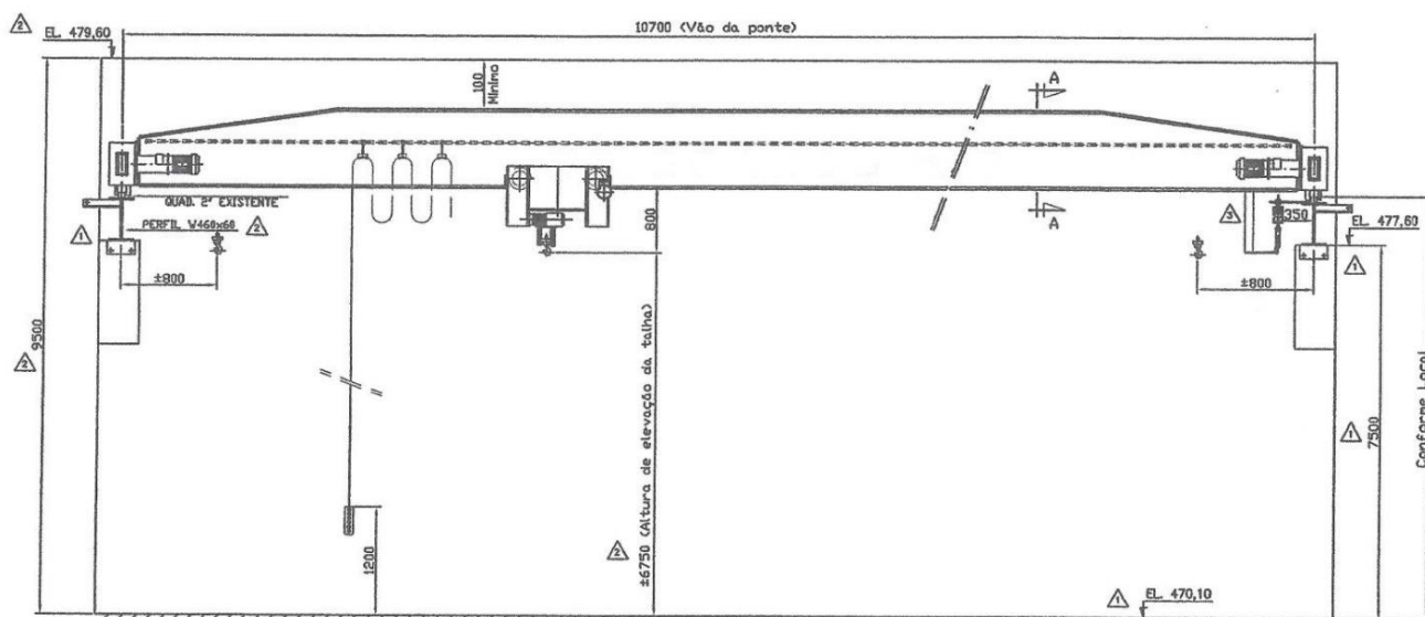
Figura 1 - Dados de projeto ponte rolante univiga apoiada – Casa de Recirculação de Lodo
